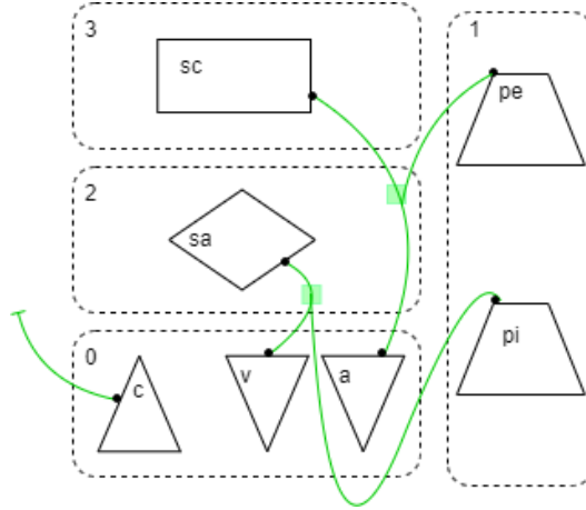
FIGURE 5.4 – Représentation graphique de l'état initial B_{exF}
