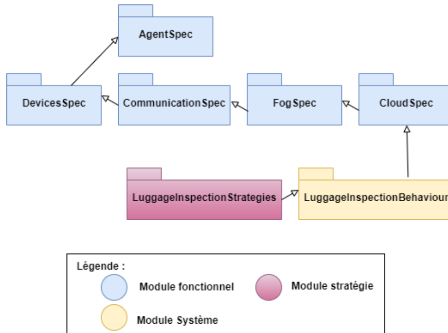
FIGURE 6.4 – Modules du système LIS dans Maude strategy
