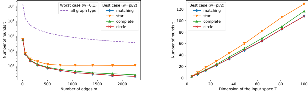
Figure C.2: Nombre de tours t nécessaires pour vérifier la condition d'arrêt (C.8) par rapport à gauche : le nombre d'arêtes m où la dimension de l'espace de \mathcal{Z} est fixée et égale à 25 et right : la dimension de l'espace de \mathcal{Z} où le nombre d'arêtes est fixé et égal à 156. Pour les deux expériences, nous les exécutons 100 fois et nous traçons le nombre moyen de tours nécessaires pour vérifier la condition d'arrêt.
