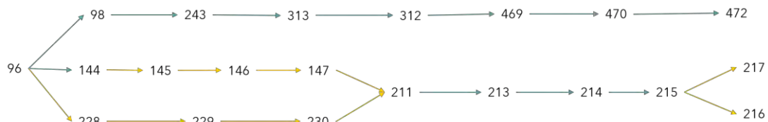
Figure 34 - Graphe de précedence des tâches de l'instance de test du critère de Choquet
