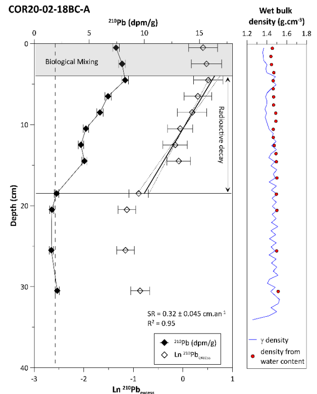
Figure 2-10. Méthode pour calculer une vitesse de sédimentation à partir de la décroissance radioactive du ^{210}\text{Pb} . Les premiers centimètres bioturbés sont exclus.
