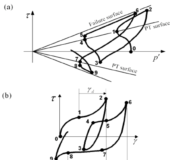
Figure 2-24. Schéma du modèle PDMY02 montrant (a) la réponse de la contrainte octaédrique \tau avec la contrainte effective p' et (b) la réponse de la contrainte octaédrique \tau avec la déformation octaédrique \gamma Yang et al. , 2003).
