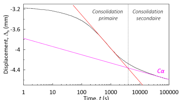
Figure 2-14. Courbe de consolidation de l'essai œdométrique COR20-02-25GC à 3.97-3.99 m de profondeur pour le palier de charge 4 kg soit ~ 220 kPa.
