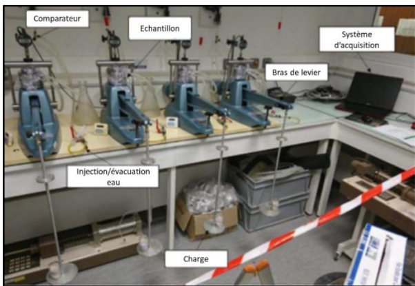
Figure 2-13. Photo du dispositif des essais œdométriques et de perméabilité au laboratoire de l'Ifremer.
