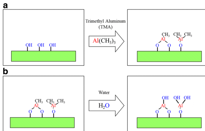
Figure 1.16 : Représentation d'un cycle de croissance d' \text{Al}_2\text{O}_3 en ALD thermique.
