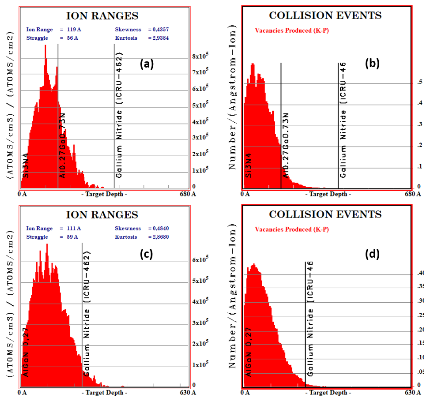
Figure 2.21 : Simulation SRIM des profils d'implantation d'ion F^+ avec cache SiN (a) et sans (c), et de collisions générant des lacunes dans la maille avec cache SiN (b) et sans (d). L'énergie d'implantation est de 7 keV.
