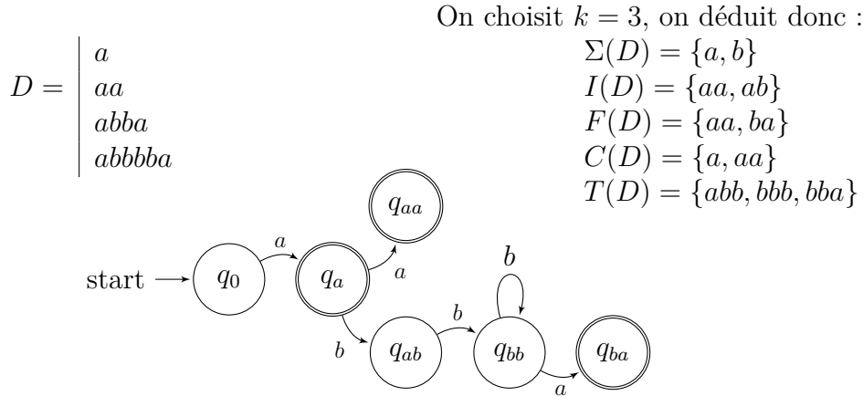
FIGURE 3.1 – Exemple de construction d'un automate k -testable
