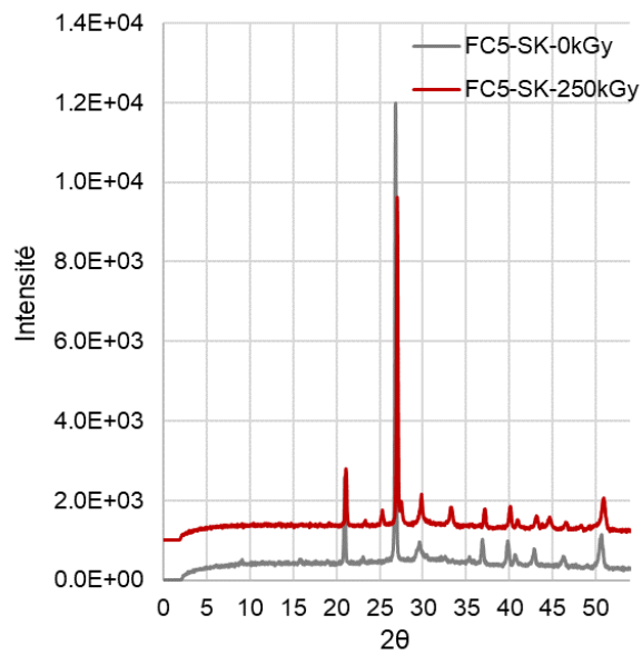
Figure 36. Diffractogrammes des coulis à base de CEM V/A adjuvantés de MG (a) et de SK (b) en fonction de la dose (0 et 250 kGy).
