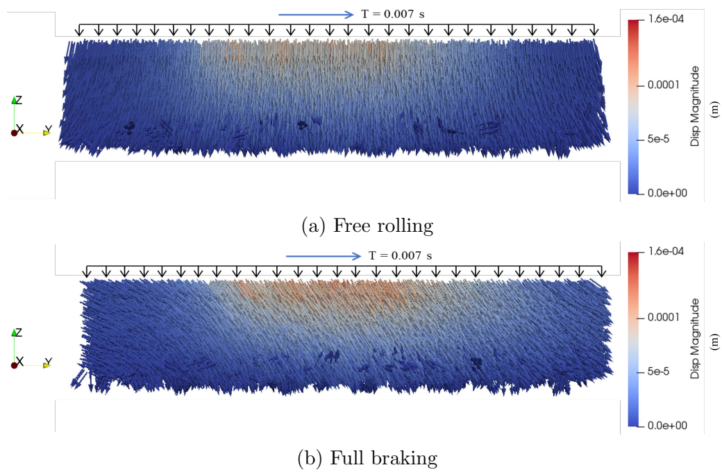
Figure 10: Distribution du déplacement des particules à 30 m/s pour différents états de roulement ( T = 0.007 \text{ s} )
