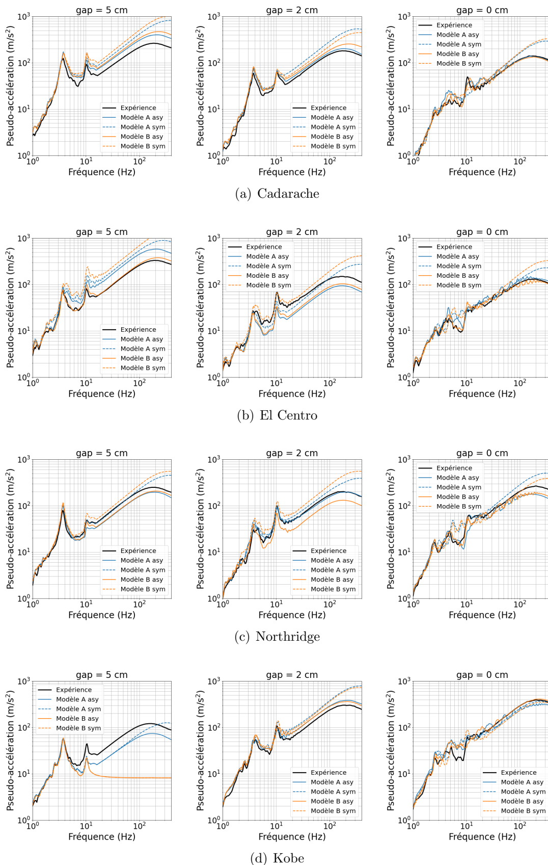
Figure 3.20: Comparaison de la pseudo-accélération au deuxième étage de la Structure 2 entre les résultats des modèles numériques (Modèles A et B, asymétriques et symétriques) et expérimentaux
