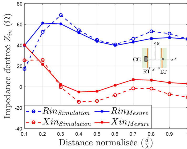
Figure 2.21 : Impédance d'entrée Z_{in} simulée et mesurée du tag LT. La résistance ( R_{in} ) et la réactance ( X_{in} ) sont tracées en fonction de la distance de séparation d (valeur normalisée) entre les deux dipôles imprimés lorsque l'antenne du tag RT est court-circuitée.
