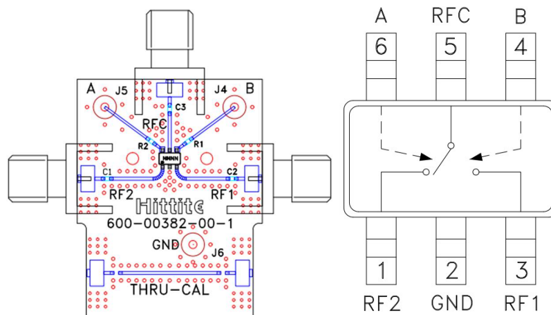
Figure 3.18 : Commutateur RF de type Hittite HMC545.
