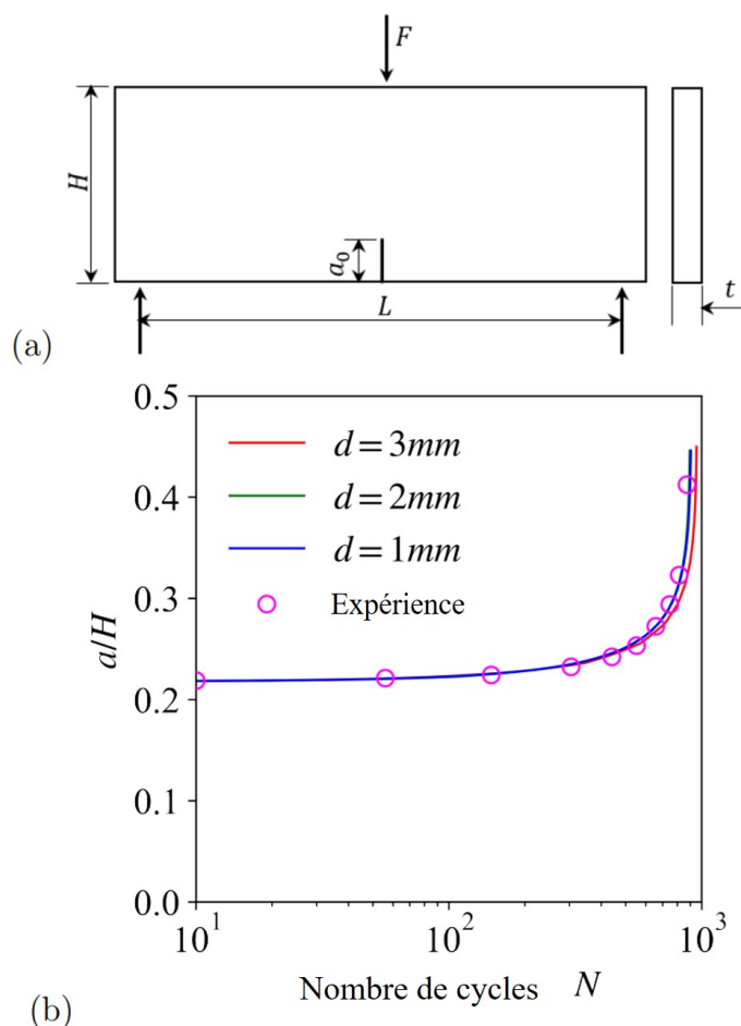
Figure 9: (a) Géométrie de la poutre en flexion trois points. (b) Evolution du rapport de longueur de fissure a/H en fonction du nombre de cycle N . Comparaison entre les résultats des essais et la simulation DEM.
