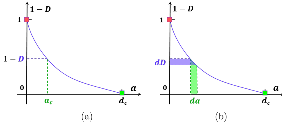
Figure 7: Transformations (a) entre a_c et D , (b) entre da et dD .
