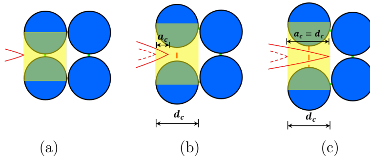
Figure 1: (a) Pointe de fissure au voisinage d'un contact et avec propagation de la fissure de (a) à (b) puis à (c), sa trajectoire pendant la rupture du contact est décrite par la variable a_c ( 0 \leq a_c \leq d_c ).
