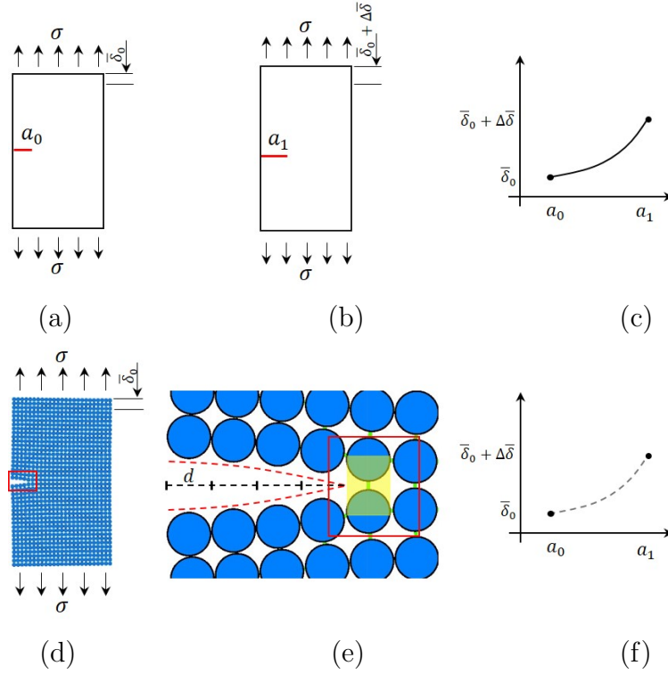
Figure 2: (a) Plaque élastique avec fissure initiale a_0 sous contrainte \sigma , déplacement résultant \bar{\delta}_0 (b) effet d’une croissance de fissure (de a_0 à a_1 ) sur les déplacements en fonction de la longueur de la fissure, (c) évolution du déplacement. (d) échantillon DEM correspondant, (e) zoom de la longueur propagée (d), et (f) évolution correspondante des déplacements en fonction de la longueur de la fissure.
