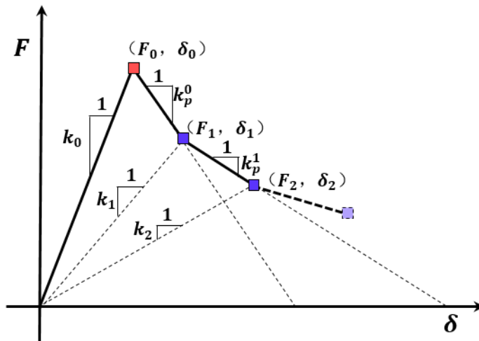
Figure 6: Description schématique de la séparation non-linéaire par traction de contact.
