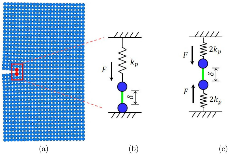
Figure 3: Description schématique de la relation mécanique entre le contact à la pointe de la fissure et les particules voisines. (a) Plaque pré-fissurée et (b) son comportement élastique simplifié près de la pointe de la fissure, où k_p représente la rigidité du matériau entourant la pointe de la fissure, F et \delta sont la force et le déplacement de contact, (c) une description plus intuitive de (b).
