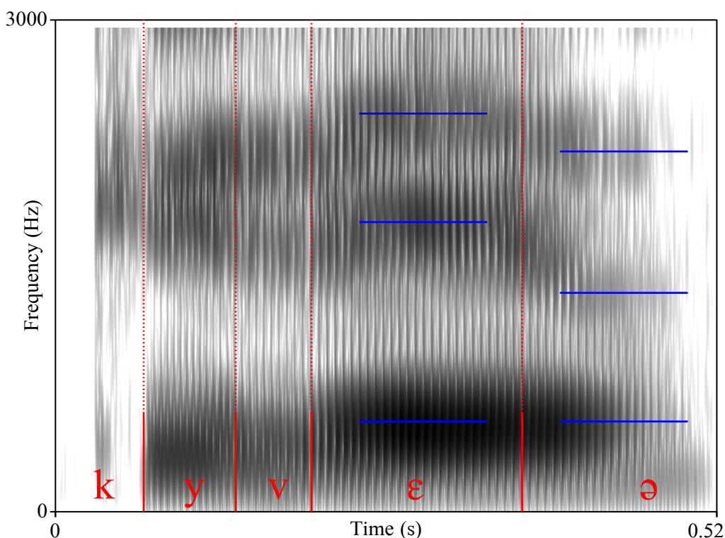
FIGURE 5.7 – Spectrogramme de cuvère "abri" (I 10 ) : le segment final, gouverné par /E/ a toutes les caractéristiques d'un vocoïde central. Outre la facile identification de ses formants, cette réalisation se distingue de la réalisation d'une rhotique par sa durée d'émission, bien supérieure à celle de [r].
