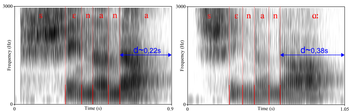
FIGURE 5.1 – Spectrogrammes comparés des s'es n-anat 1 s'en est allé (gauche) et s'es n-anaa 2 "elle s'en est allée" (droite), formes obtenues auprès de l'I 2 .
