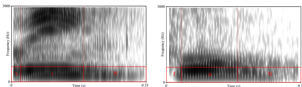
FIGURE 5.5 – Spectrogrammes des formes (ɔ) vint "vingt" (gauche) et font "sourcé" (droite). Dans les deux cas, à l'affaiblissement des formants des voyelles, succède un signal nasal (caractérisé par un bruit basse fréquence) dont la résonance est indéterminée.
