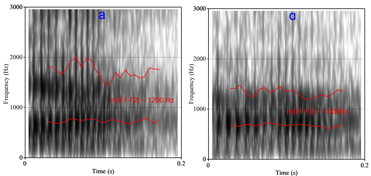
FIGURE 5.2 – Formants des voyelles toniques /a/ prise dans s'es n-ana[sEn5"na] (à gauche) et s'es n-ana[sEn5"nA:] (à gauche). Les courbes rouges indiquent la position des formants F 1 et F 2 (extraction brute de Praat). L'abaissement des formants est net dans le cas de la voyelle longue phonologique.
