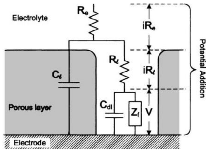
Figure II.4 : Circuit électrique équivalent pour l'impédance d'une électrode recouverte d'une couche poreuse [9]. R_e : résistance d'électrolyte, R_i : résistance dans les pores, C_t : capacité du film, C_{dl} : capacité double couche, Z_f : impédance faradique.
