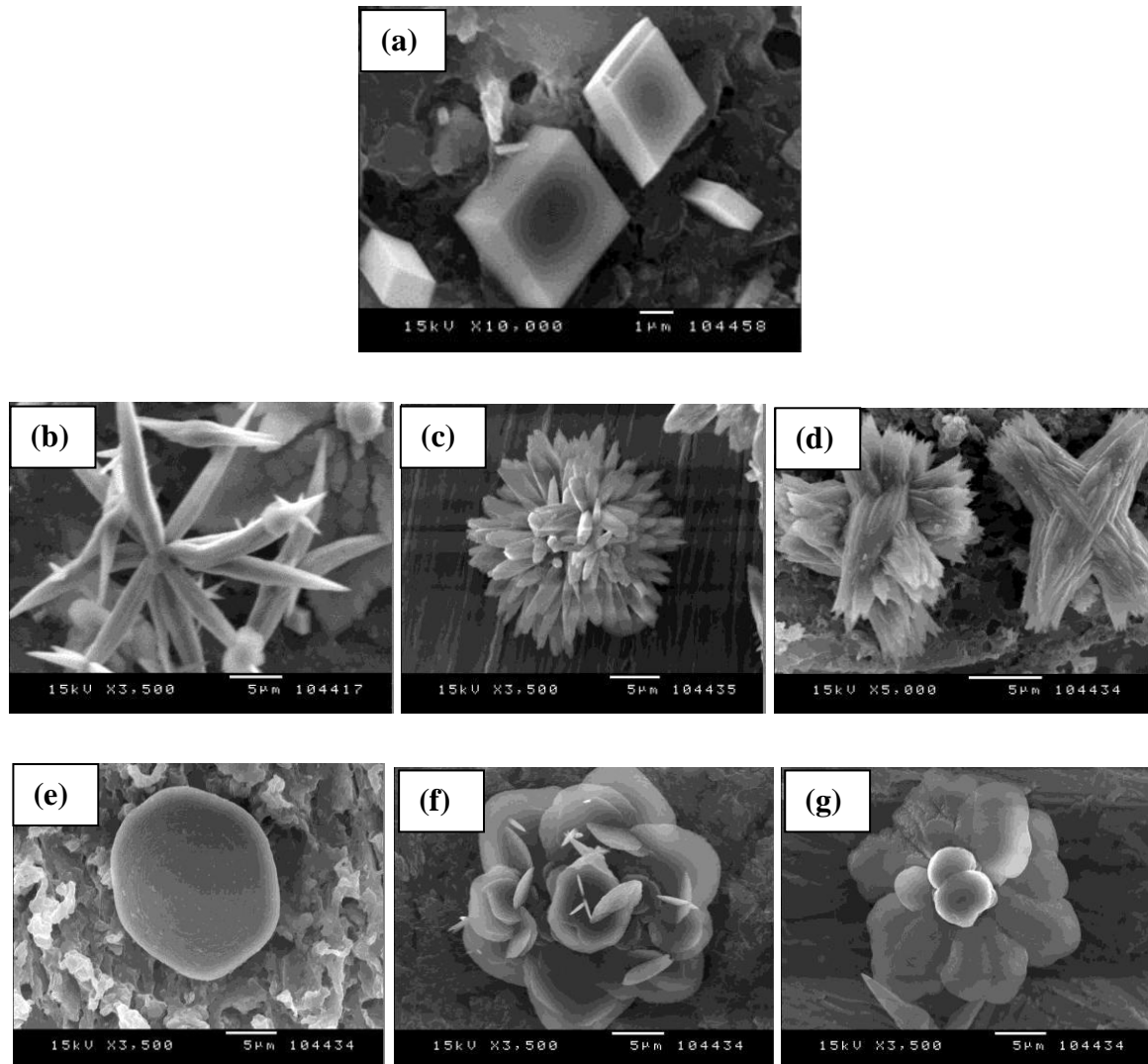
Figure I. 10 : Photos MEB, issues de la thèse Elfil, des différentes formes cristallines du carbonate de calcium : (a) calcite, (b, c, d) aragonite, (e, f, g) vaterite [40].
