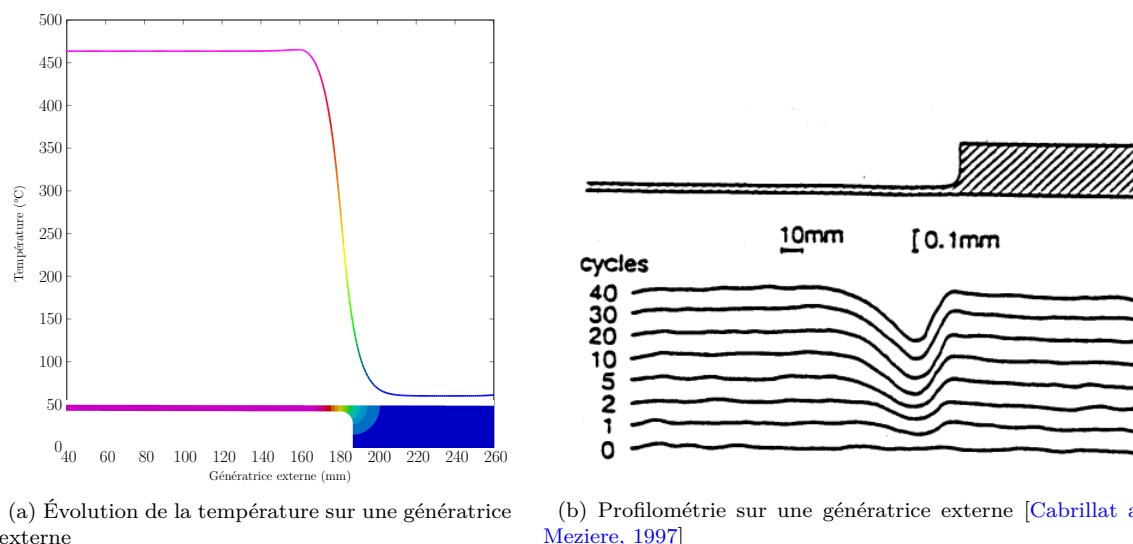
FIGURE III.3 – Principe de l'essai COTHAA
