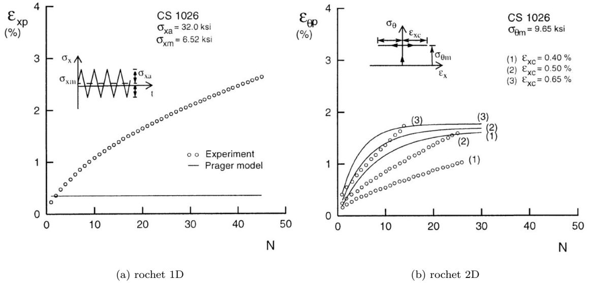
FIGURE II.5 – Réponse du modèle de Prager pour des essais de déformation progressive [Bari and Hassan, 2000]
