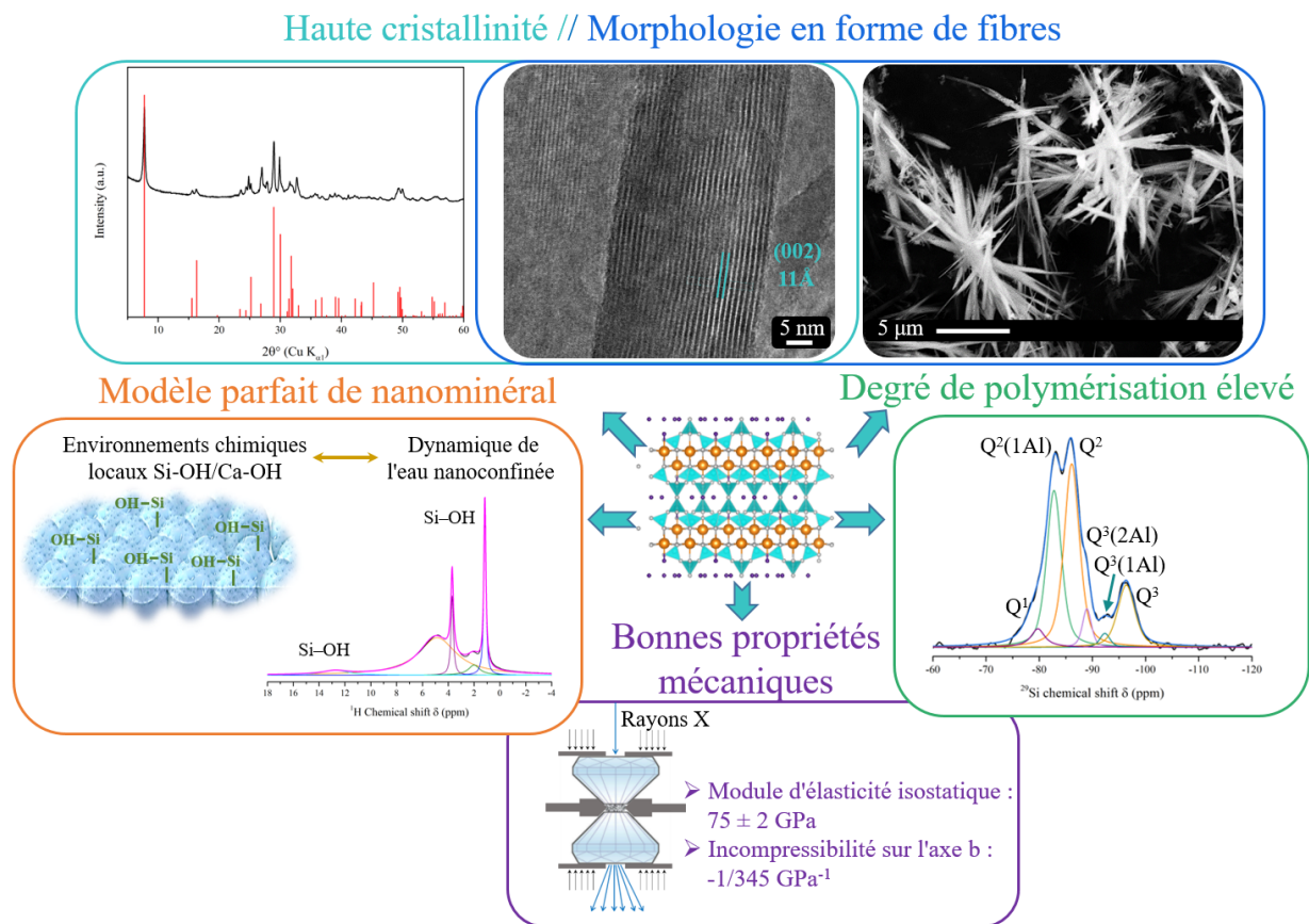
Figure 2: Schéma représentatif des propriétés physico-chimiques de la tobermorite synthétisée dans l'eau supercritique en 8 s.
