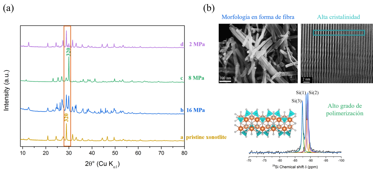
Figure 8: (a) Diagramas de difracción de rayos X de muestras sintetizadas durante la deshidratación hidrotermal a 500 °C durante 1 h a diferentes valores de presión: 16 MPa, 8 MPa y 2 MPa. (b) Diagrama representativo de las propiedades fisicoquímicas de la wollastonita sintetizada a 500 °C y 8 MPa.
