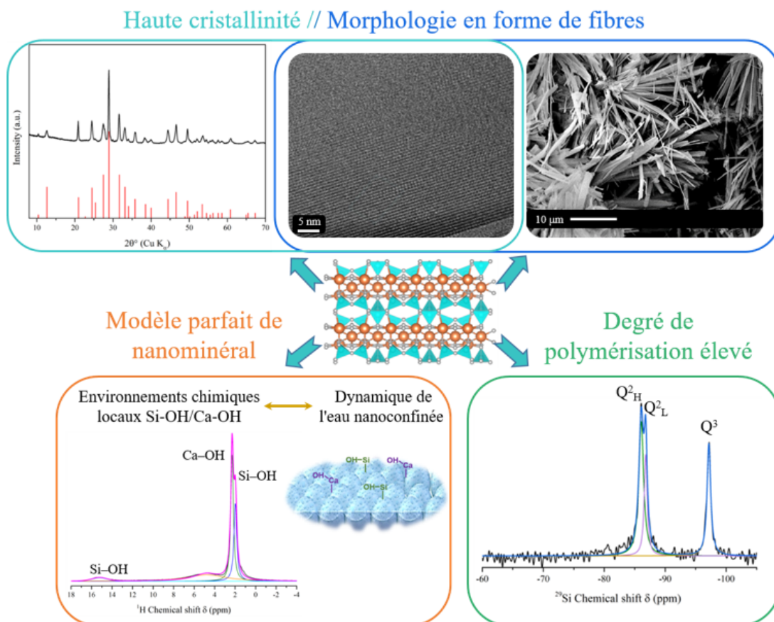
Figure 1: Schéma représentatif des propriétés physico-chimiques de la xonotlite synthétisée dans l'eau supercritique en 7 s.
