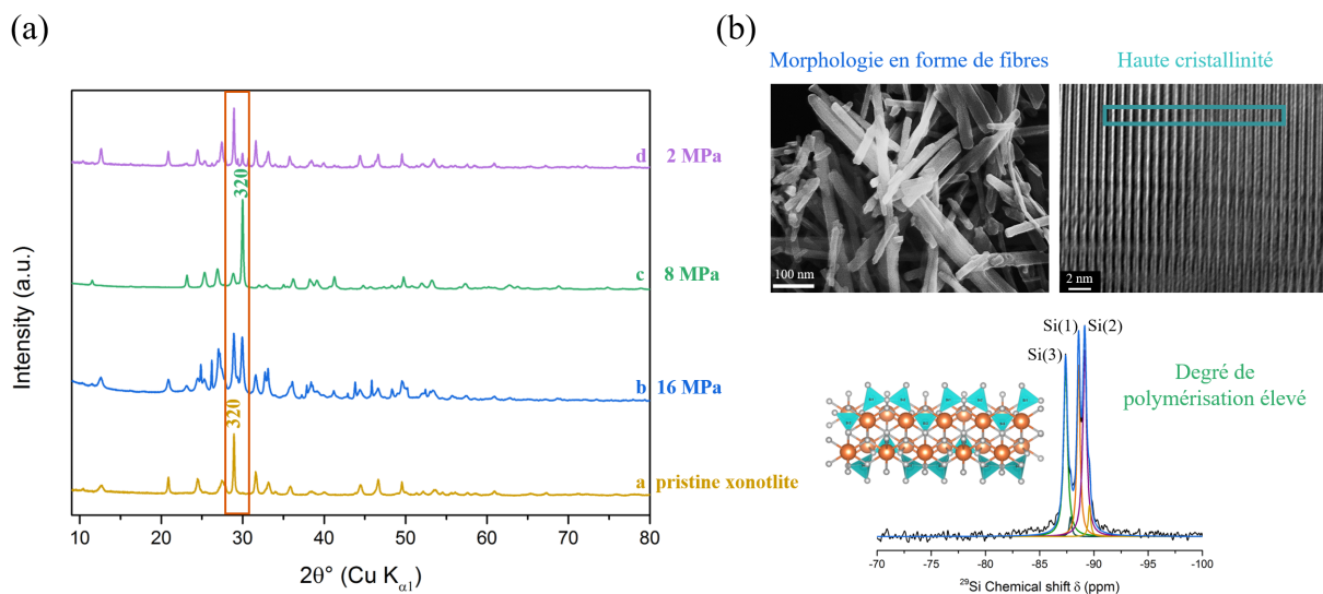
Figure 4: (a) Diagrammes de diffraction des rayons-X des échantillons synthétisés lors de la déshydratation hydrothermale à 500 °C pendant 1 h à différentes valeurs de pression: 16 MPa, 8 MPa et 2 MPa. (b) Schéma représentatif des propriétés physico-chimiques de la wollastonite synthétisée à 500 °C et 8 MPa.
