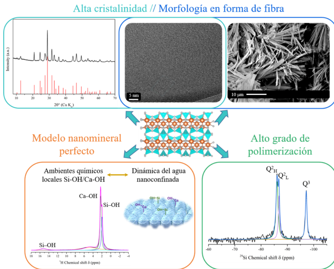
Figure 5: Diagrama representativo de las propiedades fisicoquímicas de la xonotlita sintetizada en agua supercrítica en 7 s.
