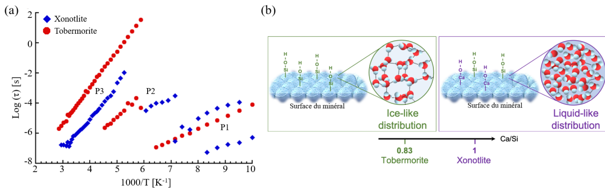
Figure 3: (a) Dépendance en température des temps de relaxation liés à la dynamique observée dans la tobermorite (en rouge) et la xonotlite (en bleu). (b) Représentation schématique de la corrélation entre la structure chimique de la xonotlite et de la tobermorite et son effet sur la dynamique de l'eau nanoconfinée, basée sur les résultats de ce travail.
