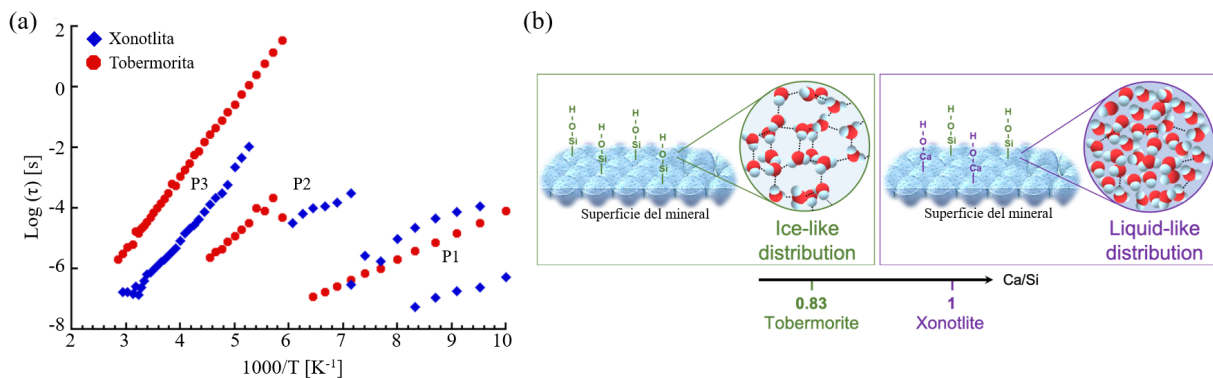
Figure 7: (a) Dependencia de la temperatura de los tiempos de relajación ligados a la dinámica observada en tobermorita (en rojo) y xonotlita (en azul). (b) Representación esquemática de la correlación entre la estructura química de la xonotlita y la tobermorita y su efecto sobre la dinámica del agua nanoconfinada, basada en los resultados de este trabajo.
