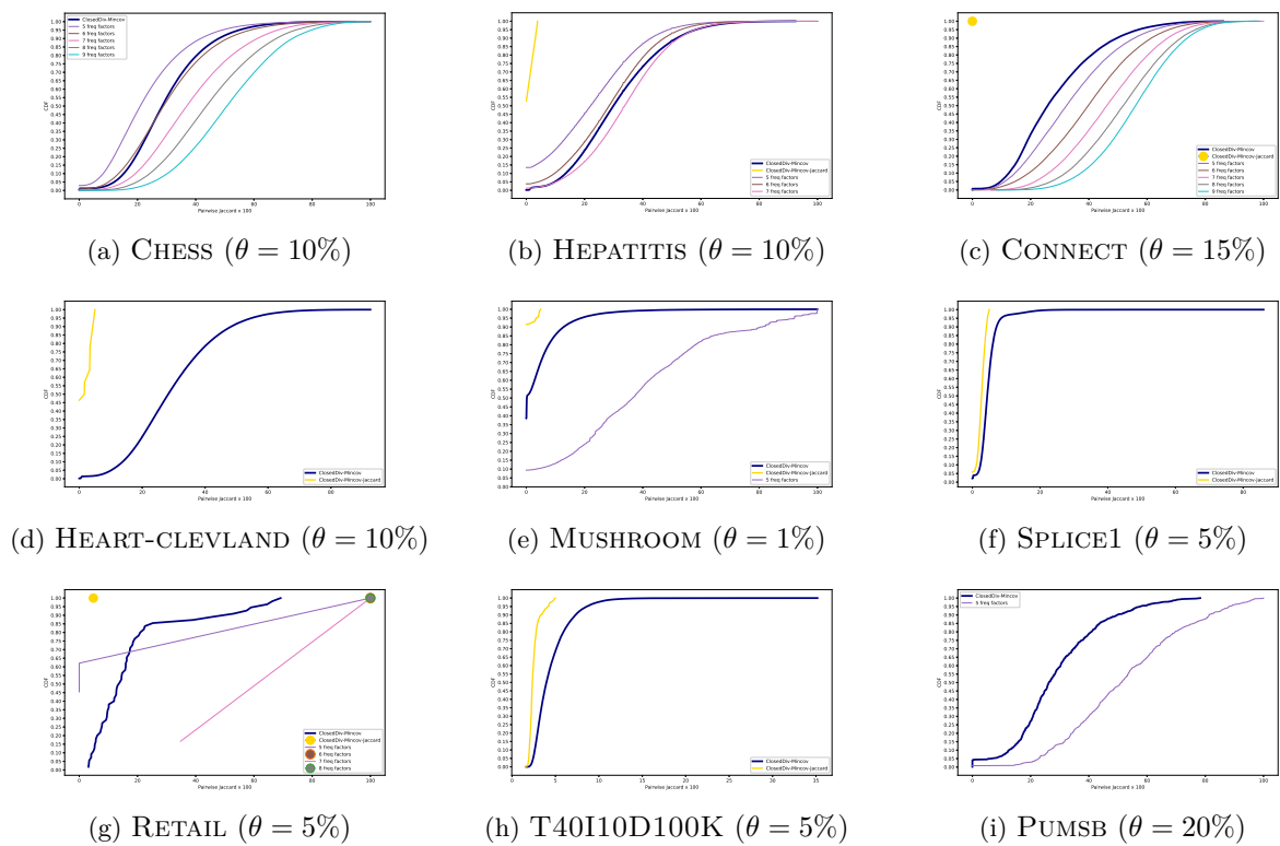
FIGURE A.6 – Analyse de la redondance dans les ensembles de motifs de CLOSEDDIV et CFTP. Nous utilisons ici des facteurs de fréquence c \in \{5, 6, 7, 8, 9\} .
