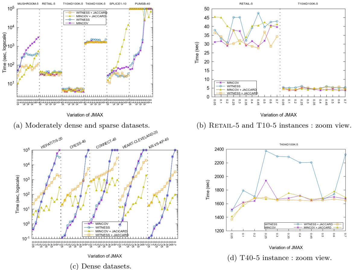
FIGURE 5.8 – Comparaison des temps d'exécution de CLOSEDIV-MINCOV et CLOSEDIV-WITNESS avec et sans test de la valeur de Jaccard
