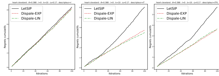
(a) HEART-CLEVELAND : regrets cumulatifs.
