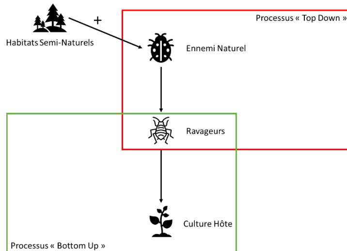
Figure 7 - Représentation simplifiée des processus « Bottom Up » et « Top Down ». La régulation bottom-up est la régulation par la base de la chaîne alimentaire ou du réseau trophique par la disponibilité en ressource alimentaire. La régulation top-down s'axe sur la prédation et ses effets sur les populations proies.
