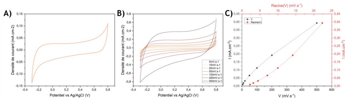
Figure IV.12 : Cyclage CV des FdC+ \text{Al}_3\text{@SiNWs} en milieu \text{Na}_2\text{SO}_4 0,2 M A) à 20 \text{ mV}\cdot\text{s}^{-1} , B) en fonction de la vitesse balayage croissante C) Représentation de la densité de courant en fonction de la vitesse de balayage ou de sa racine.
