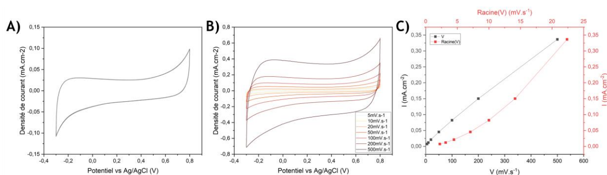
Figure IV.11 : Cyclage CV des FdC+Si-2D en milieu \text{Na}_2\text{SO}_4 0,2 M A) à 20 \text{ mV}\cdot\text{s}^{-1} , B) en fonction de la vitesse balayage croissante C) Représentation de la densité de courant en fonction de la vitesse de balayage ou de sa racine.
