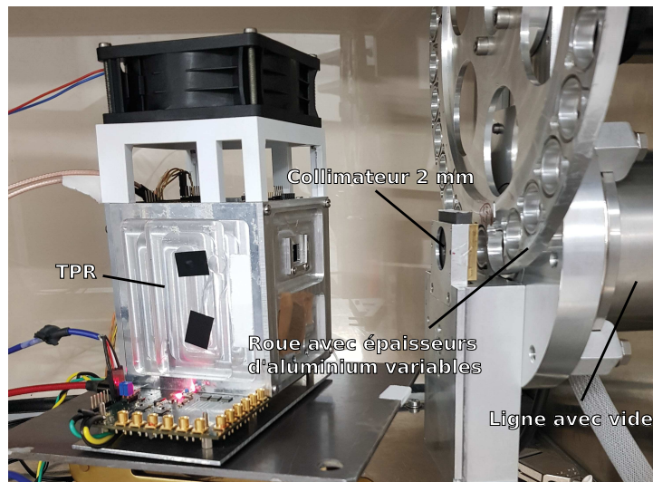
FIGURE 2.5 – Photo d'une expérience avec le TPR à l'accélérateur Cyrécé. Le détecteur est positionné à l'extrémité de la première ligne de faisceau, avec la roue et un collimateur de 2 mm.
