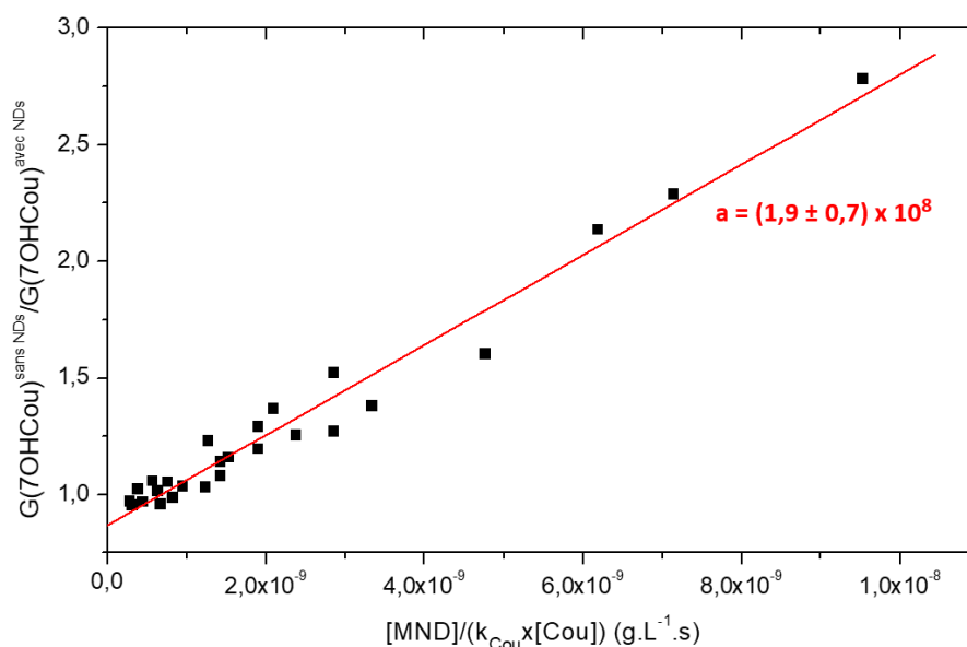
Figure V-5 : Ratio des rendements de formation de 7-OH Cou sans et avec NDs en fonction du produit [MND]/(k_{Cou} \times [Cou]) . En rouge sont indiquées la pente de la régression linéaire ainsi que l'erreur sur la régression.
