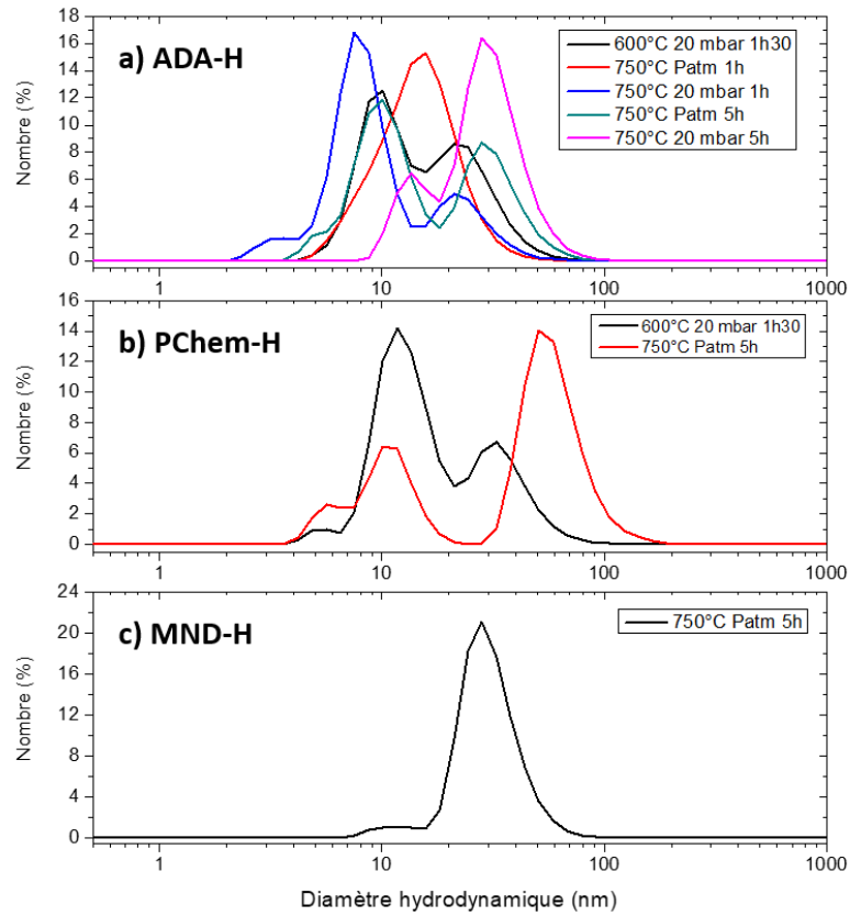
Figure II-21 : Distribution des diamètres hydrodynamiques en nombre des particules : a) ADA-H, b) PChem-H, c) MND-H. Concentration d'analyse : 0,5 mg.mL -1 . Distributions moyennées sur 30 spectres.
