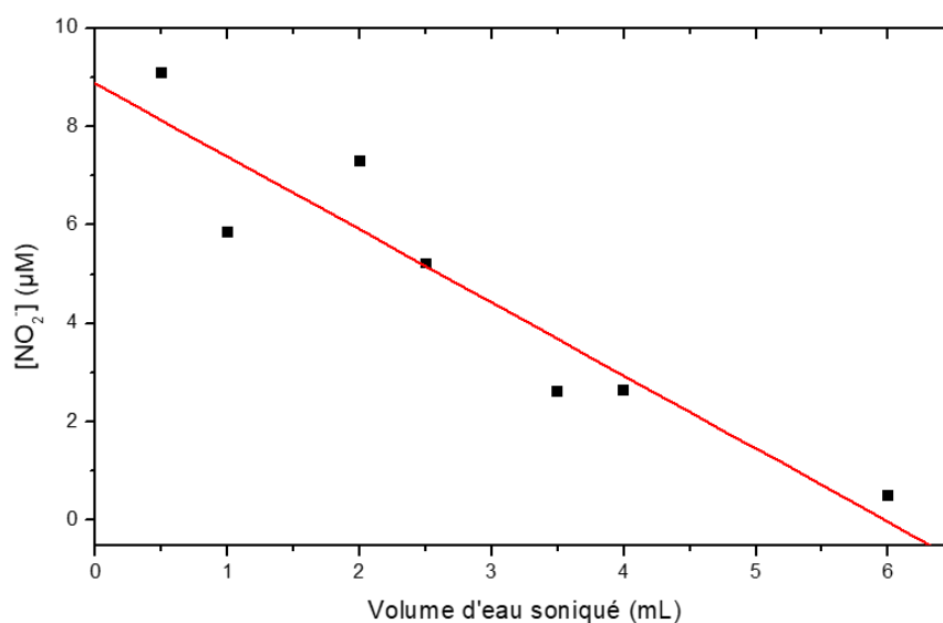
Figure II-31 : Concentration d'ions nitrite en fonction du volume d'eau soniqué.
