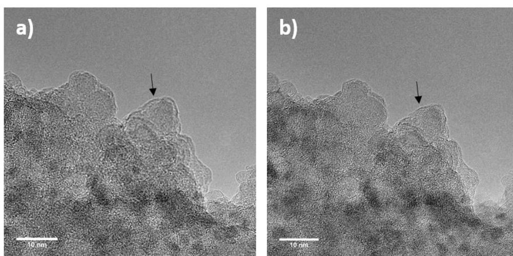
Figure III-13 : Observations MET-HR d'une zone avec des particules recuites à 1100°C sous vide: a) Défocus au Scherzer étendu et b) Plan focal. Les flèches noires pointent la monocouche organisée de C-sp^2 générée.
