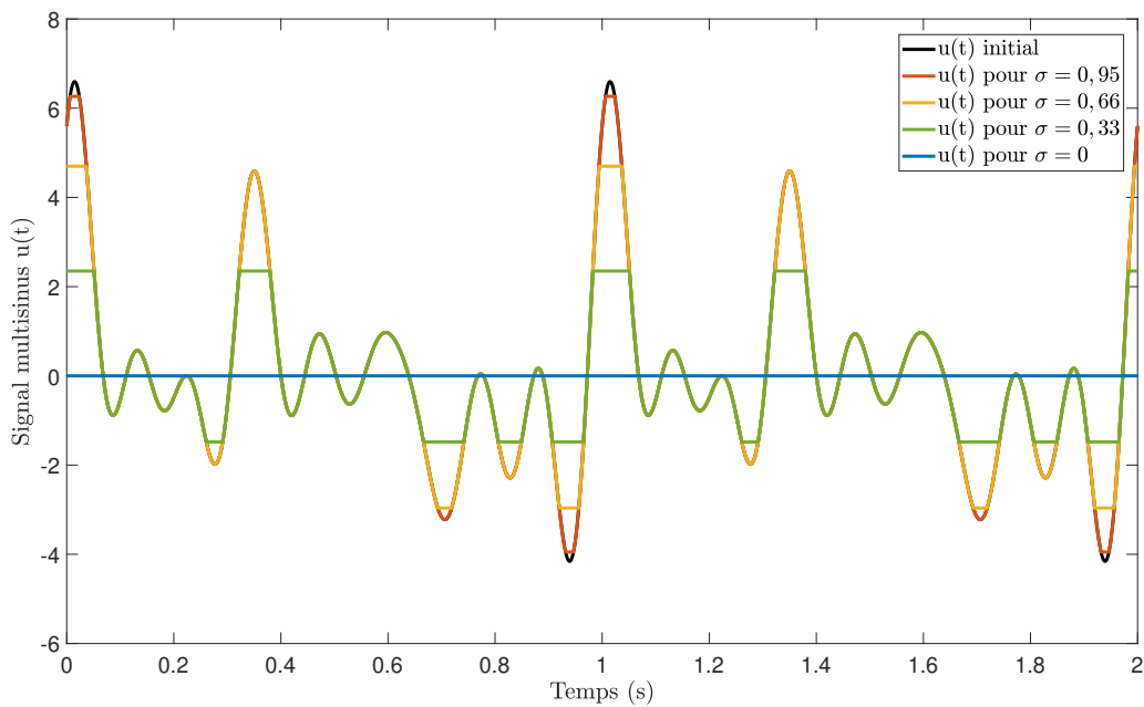
FIGURE 4.2 – Variation du niveau d'écrtage en fonction de \sigma .
