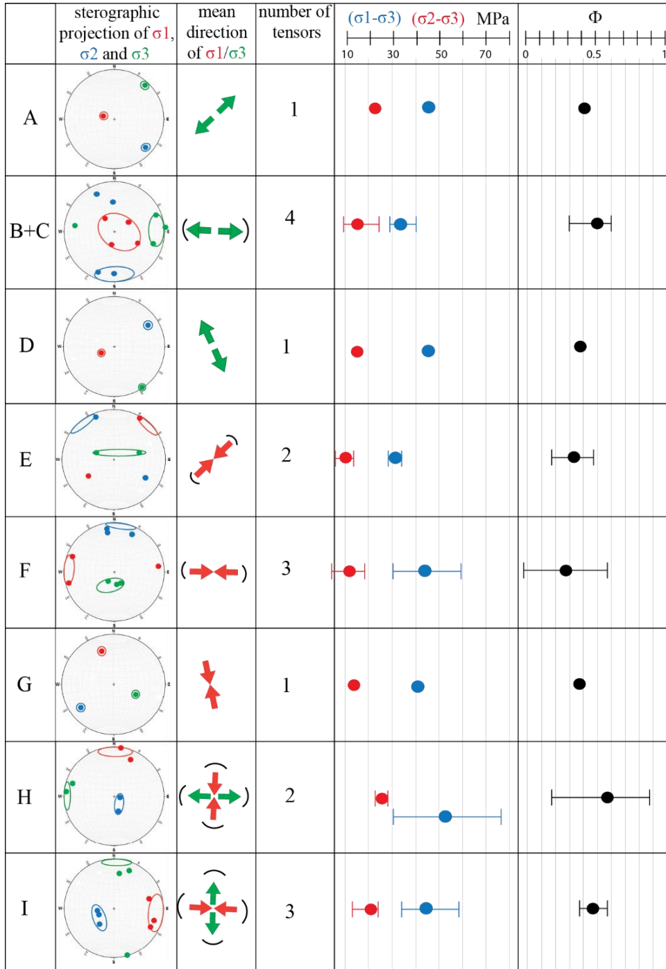
Figure 16: Groupes de tenseurs de contrainte obtenus par l'inversion des macles de la calcite. Chaque groupe de tenseurs (A à I) est caractérisé par une projection stéréographique montrant l'orientation des axes des contraintes principales (rouge pour \sigma_1 , bleu pour \sigma_2 et vert pour \sigma_3 ) et la représentation de la direction moyenne des contraintes principales horizontales sous forme de flèches (rouge pour \sigma_1 , vert pour \sigma_3 , en vue cartographique). Le nombre d'échantillons pour chaque groupe de tenseurs est indiqué ainsi que les valeurs moyennes des magnitudes des différentiels de contrainte pour chaque groupe : en bleu ( \sigma_1 - \sigma_3 ) ; en rouge ( \sigma_2 - \sigma_3 ) et en noir la valeur moyenne du rapport \Phi .
