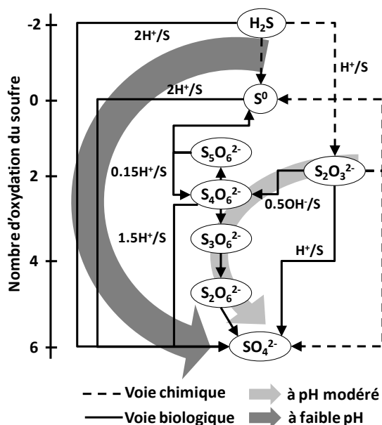
Figure 7: Oxydation des composés sulfurés au cours de la succession bactérienne (adapté de Islander et al., 1991).
