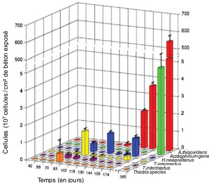
Figure 11: Evolution en nombre du type de cellules sulfo-oxydantes détectées par des analyses FISH réalisées par des sondes d'espèces ou de gènes spécifiques. Les barres d'erreur représentent l'erreur standard de mesures réalisées en duplicata (Okabe et al., 2007).
