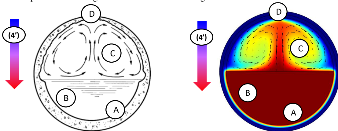
Figure 6: Schéma (adapté de Pomeroy and Boon (1990), lui-même adapté de l'agence de la protection de l'environnement des USA (USEPA, 1974)), et résultat de simulation (COMSOL multiphysics®) illustrant par les phénomènes de convection de l'air dans la canalisation (dus au gradient de température) la focalisation des flux matières dans la phase atmosphérique des canalisations gravitaires vers le sommet de la canalisation.
