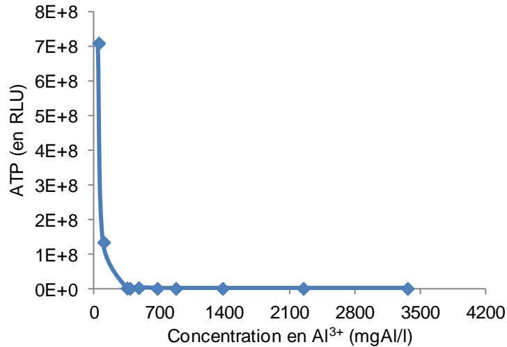
Figure 15 : mesure d'ATP totale en fonction de la concentration en aluminium total mesurée au niveau de manche creux recueillant l'eau condensée associée à des échantillons de différents mortiers disposés sur des sites réels exposés à des biodégradations avérées (Herisson, 2012)
