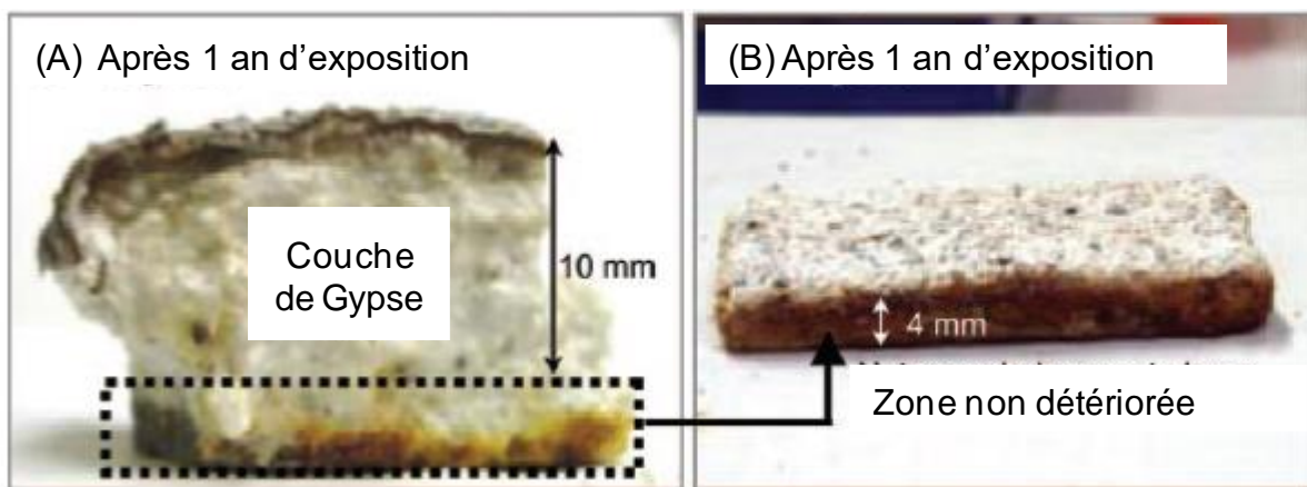
Figure 13 : Observation de la formation d'une couche de gypse en surface d'un coupon positionné dans la phase aérienne d'un regard de visite après 1 an d'exposition à des concentrations en H 2 S en phase gaz entre 20 – 30 ppm (A). La photo (B) correspond à la zone non corrodée après lessivage de la surcouche de gypse formée présentée à la photo (A) – les coupons neufs ayant une épaisseur de 8 mm (Okabe et al., 2007).
