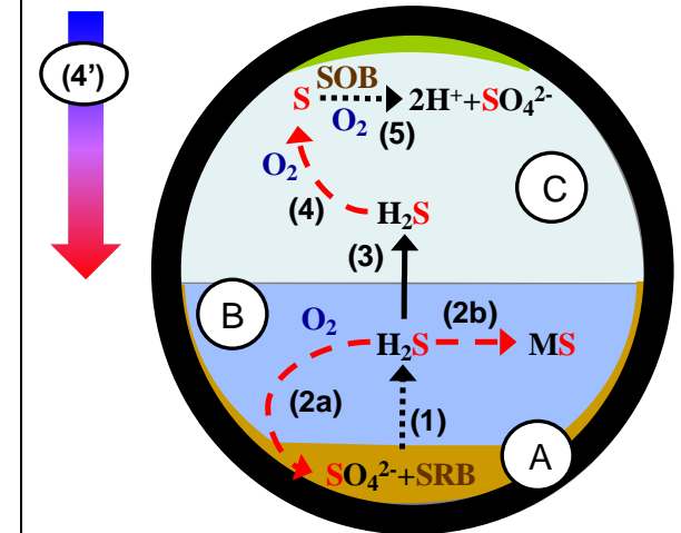
Figure 2 : Cycle du soufre dans une canalisation d'assainissement. Quatre zones particulières sont identifiées ; A : sédiment et biofilm immergé (1) production d' H_2S par des bactéries sulfato-réductrices (SRB) ; B : phase liquide dans la zone aérobie oxydation d' H_2S avec O_2 (2a) et précipitation S^{2-} avec cation divalent ( Fe^{2+} ...) (2b) ; C : Phase atmosphérique (zone aérobie) volatilisation de l' H_2S , flux matière dirigé vers le haut de la canalisation (conditionné par le gradient de température entre la paroi de la canalisation enterrée et les eaux usées collectées) ; D : Paroi canalisation (revêtement cimentaire) 5 : Zone humide → développement Biofilm ; 6 : Gradient de température ; SOB : bactéries sulfo-oxydantes ; S(X) : Composés soufrés. Adapted from (Hitvited-Jacobsen, 2002)
