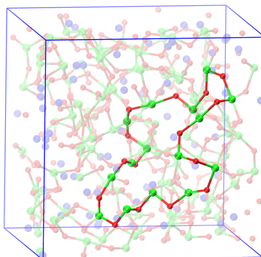
(d) Ring of size 30 in 40%- \text{TlO}_{0.5} -60% \text{TeO}_2 .
