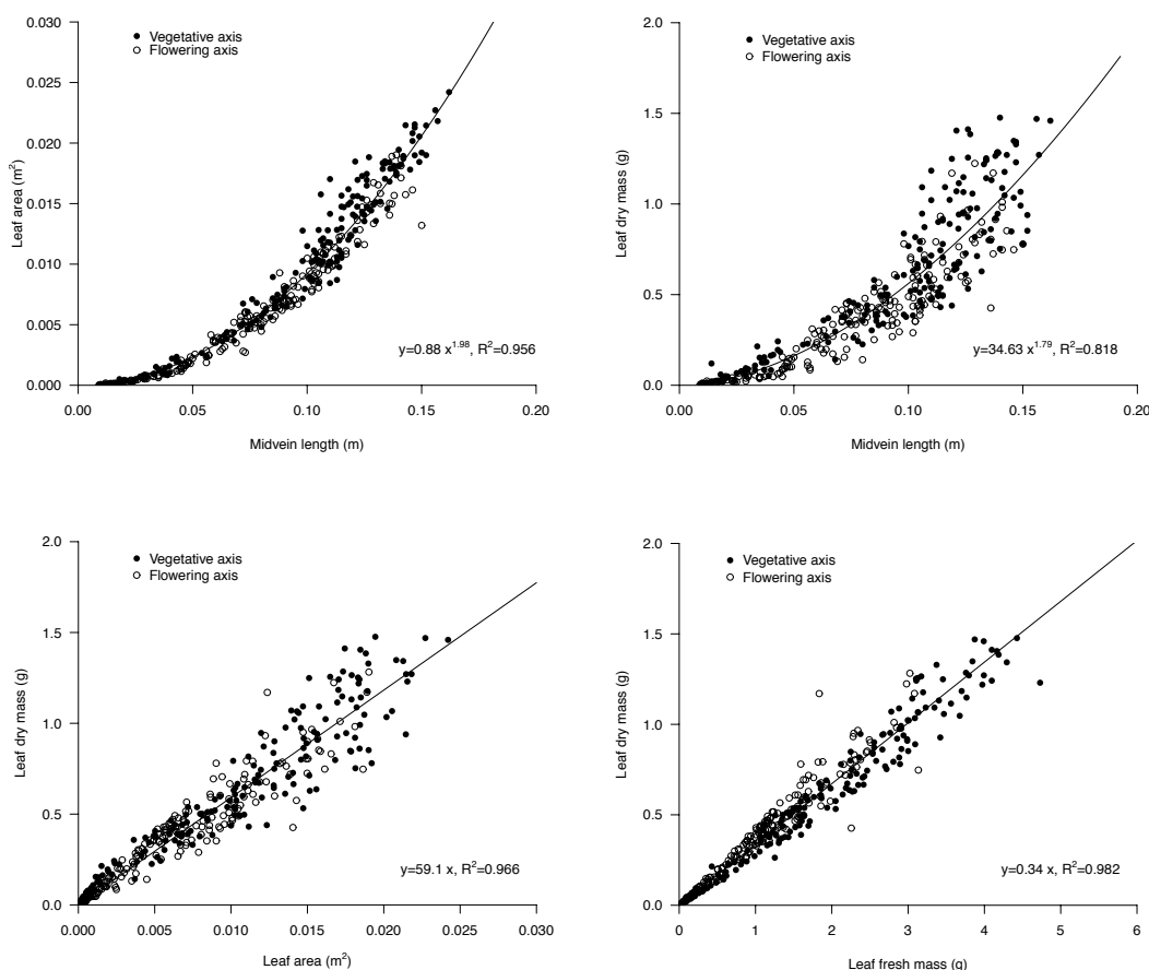
Figure 5.2 – Relations entre la surface des feuilles de Rubus alceifolius ( m^2 ) et la longueur de la nervure principale (m), et entre la masse sèche (g) et la longueur de la nervure principale (m), la surface foliaire, et la masse fraîche (g) pour les axes végétatifs et florifères.
