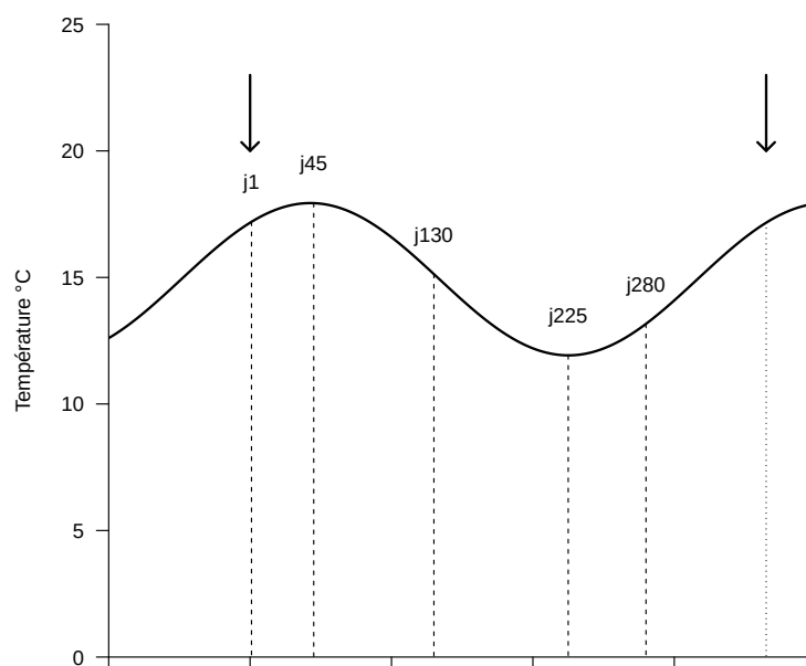
Figure 6.3 – Variations de la température quotidienne moyenne (°C) à l'altitude de 1350 m. Les jours indiqués correspondent aux dates des lâchers initiaux testées dans les simulations de la dynamique à température variable. Les deux flèches indiquent la position du 1 er janvier et du 31 décembre sur la courbe des températures.
