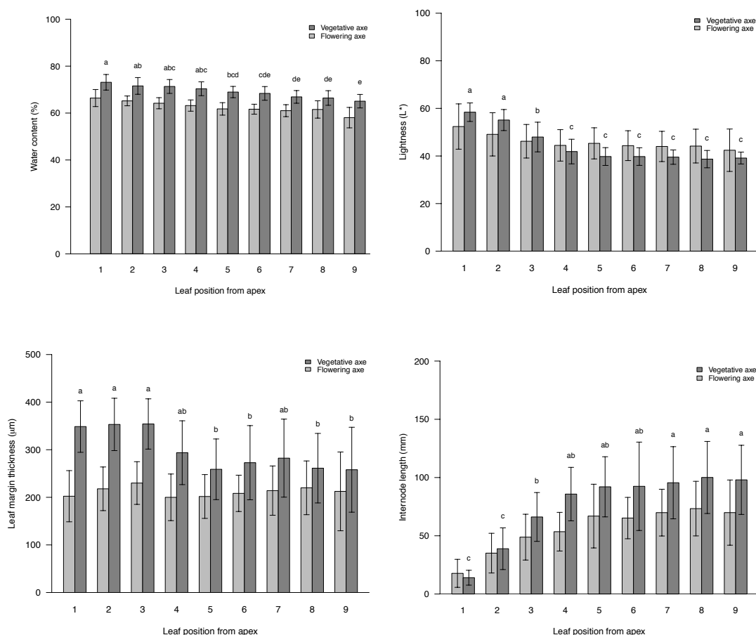
Figure 5.3 – Proportion d'eau (%), clarté (L*), épaisseur du limbe (μm) des feuilles de Rubus alceifolius et longueur des inter-nœuds (mm) selon la position de la feuille le long des axes végétatifs et florifères. Les moyennes des mesures pour les feuilles des axes végétatifs qui ne partagent pas la même lettre sont significativement différentes au test HSD de Tukey-Kramer à 5%.
