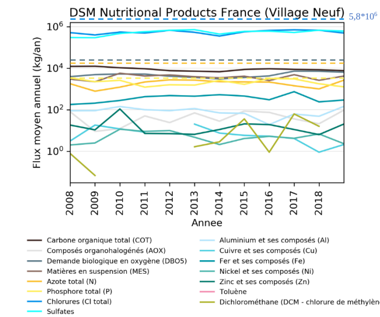
Figure 28-Evolution des rejets de DSM (DRIRE)
