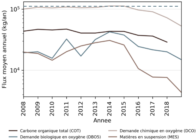
Figure 30-Evolution des rejets de Essity Opérations (BDREP)
