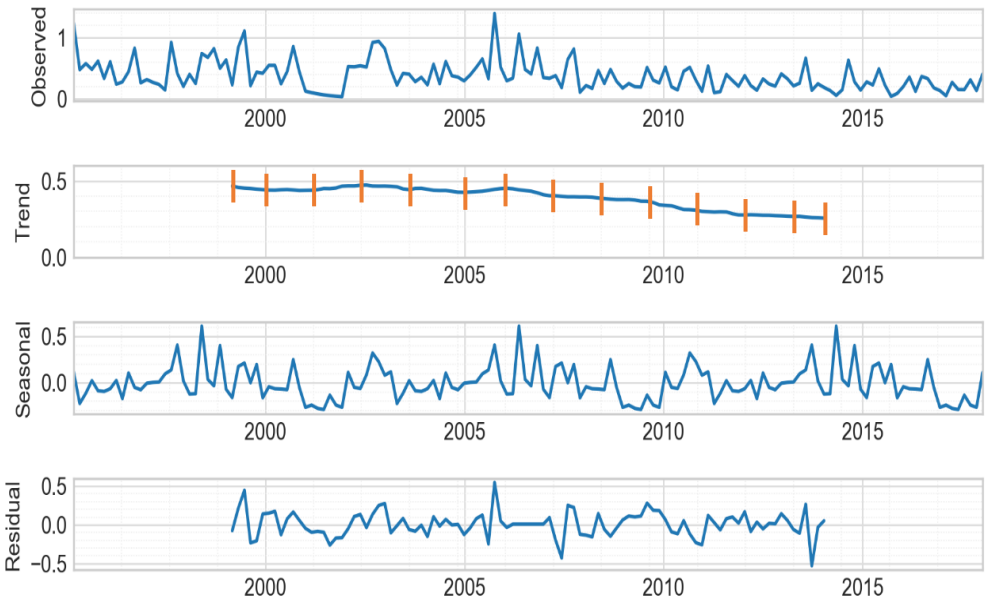
Figure 98-Décomposition en séries élémentaires et incertitudes de mesures du Plomb – (Weil-am-Rhein) en µg/l
