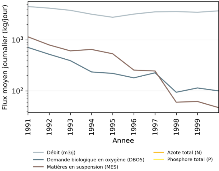
Figure 29-Evolution des rejets de Essity Opérations (DRIRE)
