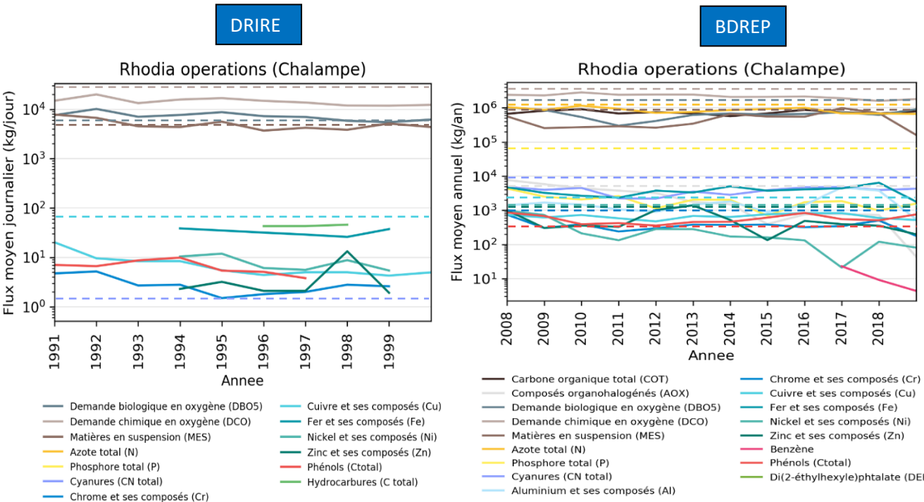
Figure 18-Evolution des rejets de Rhodia Opérations (DRIRE & BDREP)
