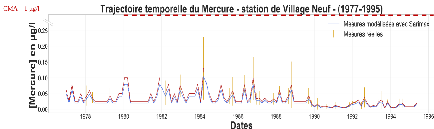
Figure 54-Exemple pour illustrer le modèle SARIMAX (1)
