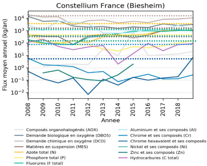
Figure 34-Evolution des rejets de Constellum France (BDREP)
