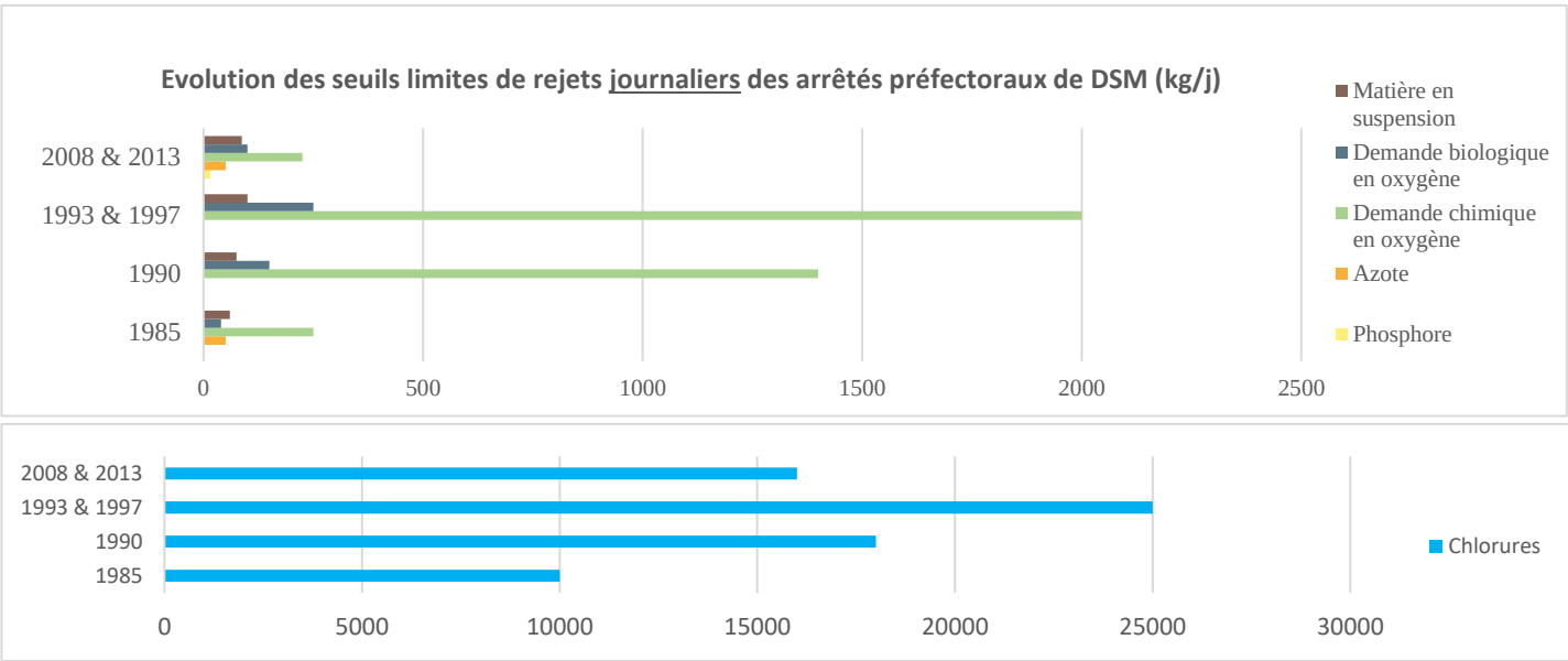
Figure 27-Evolution des seuils limites de rejets journaliers des arrêtés préfectoraux de DSM
