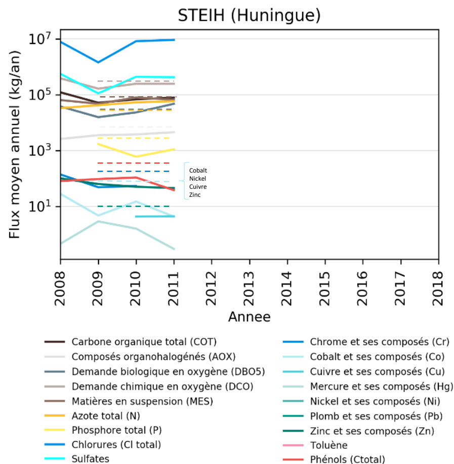
Figure 39-Evolution des rejets de la STEIH (BDREP)
