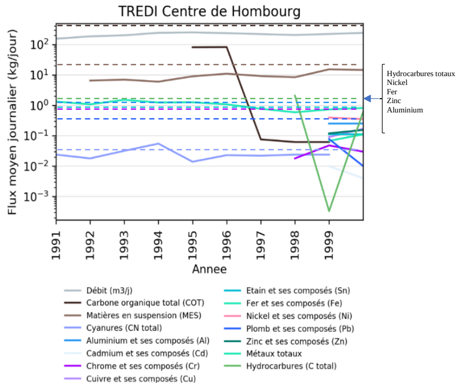
Figure 36-Evolution des rejets de Tredi (DRIRE)
