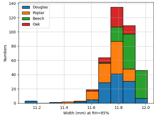
(d) Width at RH = 85%
