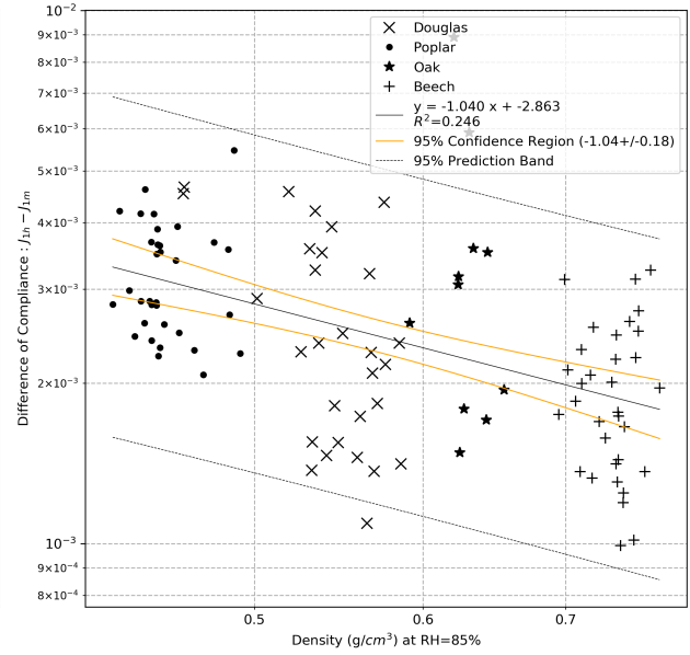
(b) J_{1h} - J_{1m}
