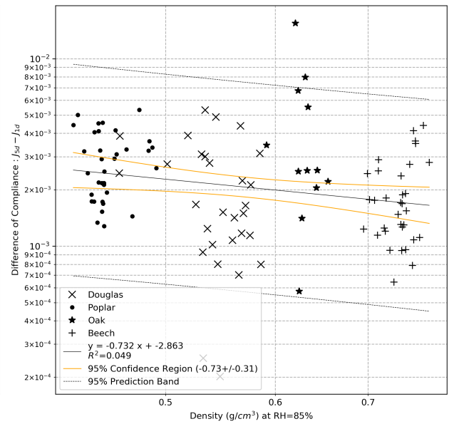
(d) J_{5d} - J_{1d}
