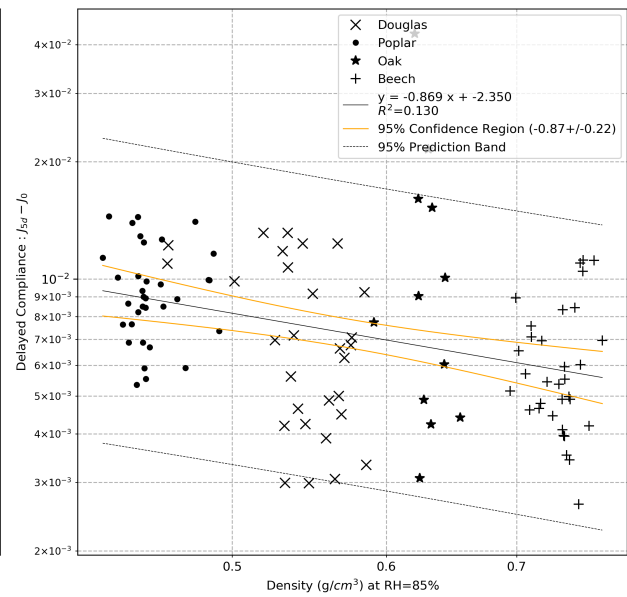
(d) J_{5d} - J_0
