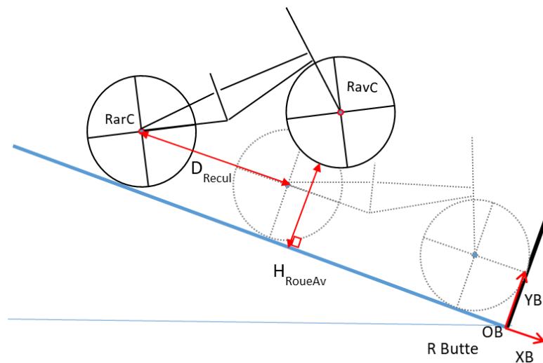
Figure 6.3: Schéma illustrant les deux paramètres de distance lors de la phase de recul du vélo: "slingshot". En pointillé le vélo en position de départ contre la grille, et en trait continu le vélo en fin de phase de recul.
