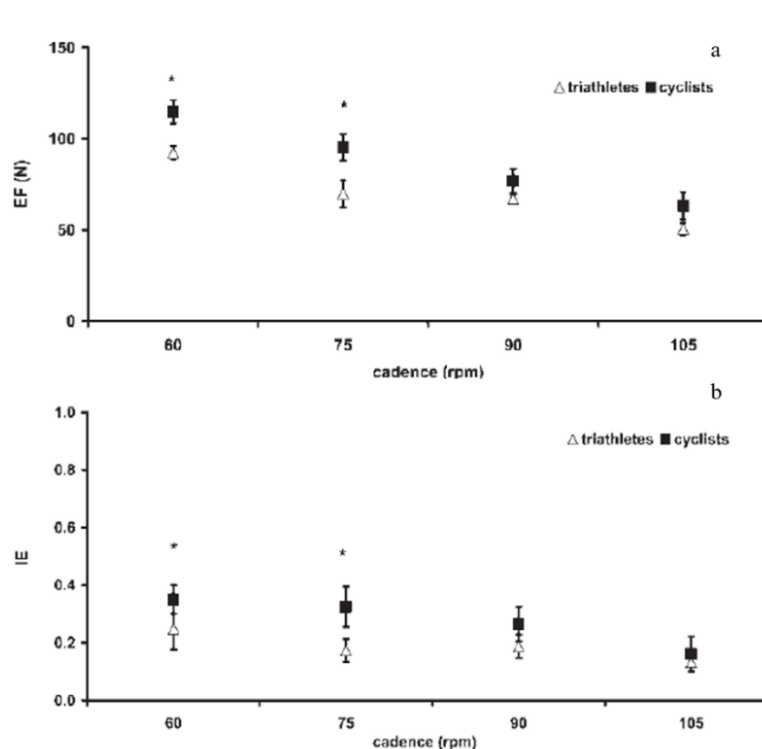
Figure 4.3: Moyenne et écart type de (a) la force efficace (EF), composante de force normale à la manivelle, et (b) l'indice d'efficacité pour des cyclistes et des triathloniens aux différentes cadences (* p < 0.05 ) (Candotti et al., 2007)
