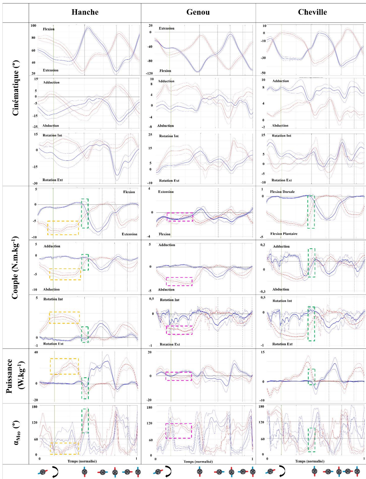
Figure 5.8: Moyenne et écart type de la cinématique (°), des moments (N.m.kg -1 ), de la puissance (W.kg -1 ) et de l'angle (°) aux articulations de la hanche, du genou et de la cheville pour le pilote P01. Les résultats sont basés sur les 6 départs de ce même pilote. Les pieds avant et arrière sont respectivement en rouge et bleu. La ligne verticale verte indique le moment où la grille tombe. Chaque illustration de pédalier en axe des abscisses indique la position angulaire approximative dans laquelle se trouve le pédalier à l'instant t .
