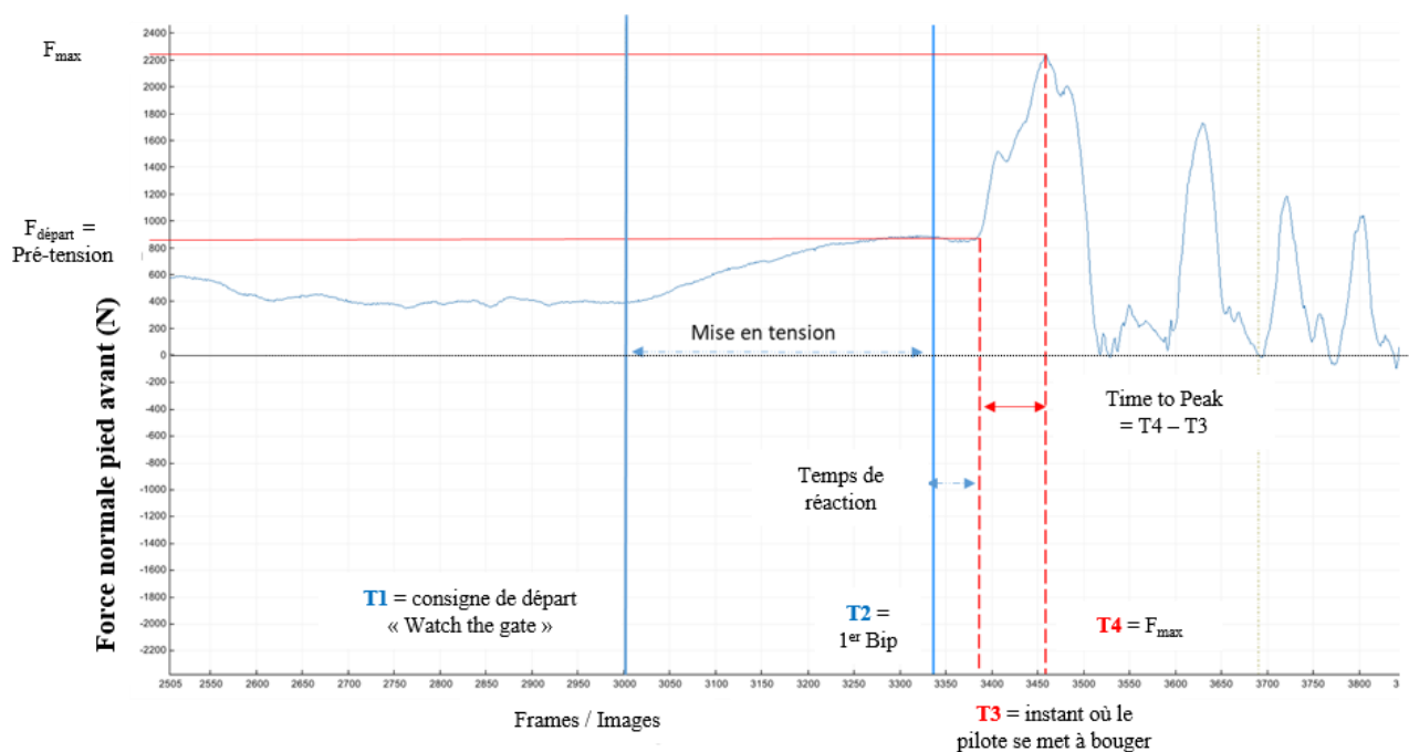
Figure 6.4: Graphique illustrant l'évolution de la force utile du pied avant (pied de départ) au cours du temps ainsi que les paramètres analysés.
