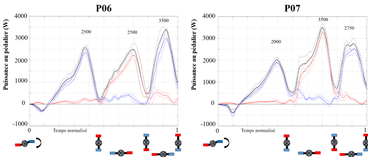
Figure 6.7: Moyenne et écart type de la puissance globale (noire) produite au pédalier par le pied avant (bleu) et le pied arrière (rouge) en W lors des trois premiers coups de pédales pour les pilotes P06 et P07.
