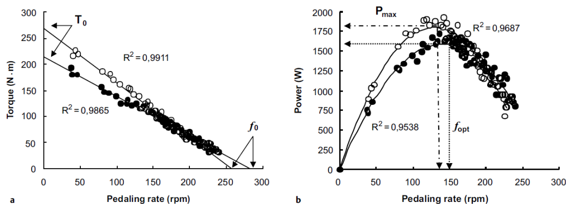
Figure 1.8: Relations couple (a) et puissance -vitesse (b) de deux athlètes, F et K, valeurs moyennées pendant la phase de descendante de la pédale obtenues de trois sprints de 5 secondes. Détermination de la puissance maximale ( P_{max} ), la cadence optimale ( f_{opt} ), de la cadence maximale ( f_0 ), et du couple maximal ( T_0 ). Athlète F : cercle plein. Athlète K : cercle vide. (Dorel et al., 2005)
