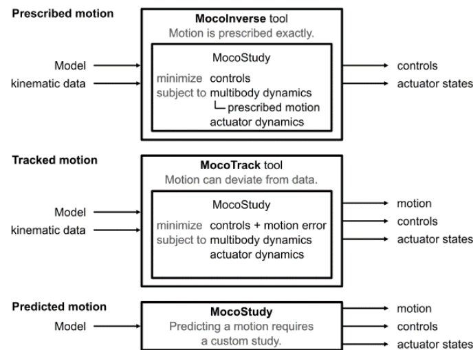
Figure 7.8: Les trois outils présents permettant la simulation par l'intermédiaire d'OpenSim Moco: MocoInverse, MocoTracked et MocoStudy. Les données d'entrées, inputs, pour la résolution sont sur la gauche de la boîte de traitement et les variables en sortie à droite (Dembia et al., 2020).
