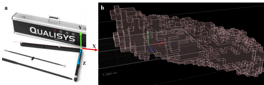
Figure 2.5: (a) Kit de calibration comprenant l'équerre et la "baguette". (b) Volume calibré sur la butte et visualisation du référentiel R_0 créé au niveau de la grille, l'axe x parallèle à l'horizontale.
