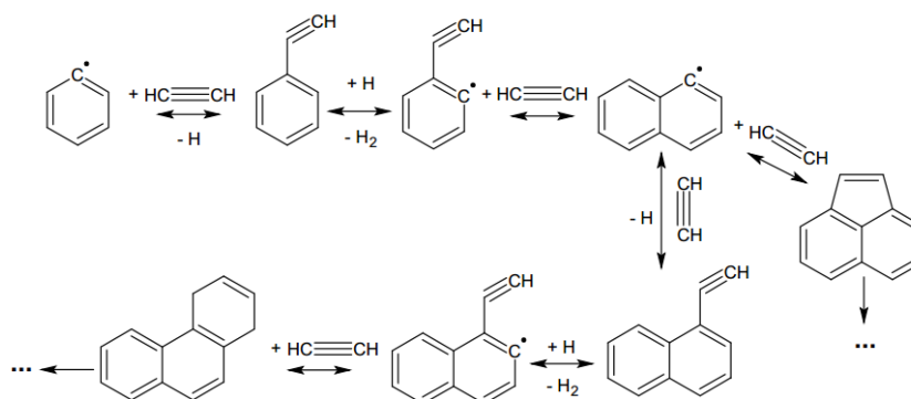
Figure 1.2 : schéma réactionnel de croissance des HAPs par le mécanisme HACA [28].
