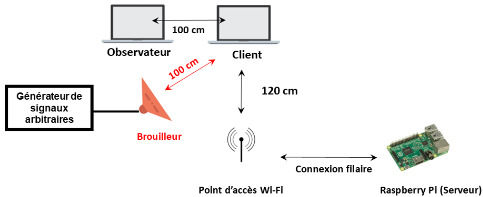
FIGURE 3.2 – La situation avec une attaque par brouillage
