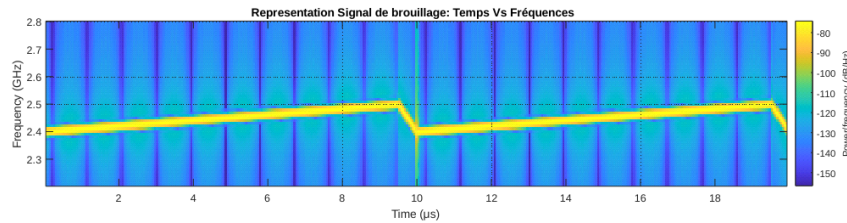
FIGURE 3.3 – Exemple de représentation du signal de brouillage
