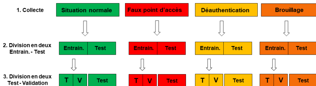
FIGURE 4.8 – Division des données
