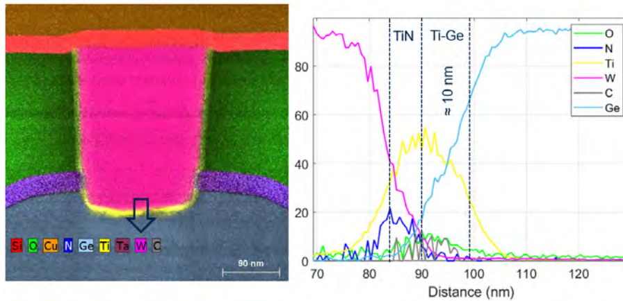
FIGURE 5.15 – Analyse TEM-EDX d'un contact Ti/p-Ge formé avec un recuit à 850 °C pendant 30 s.
