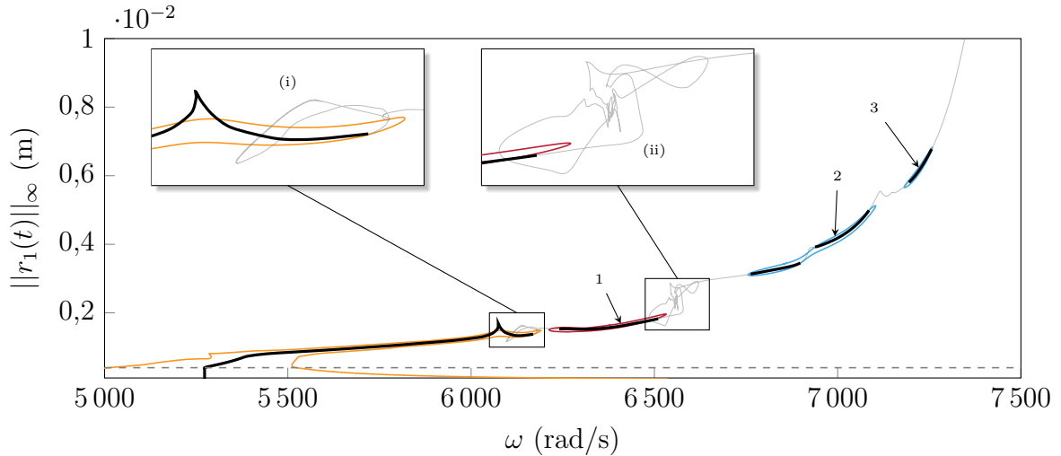
FIGURE V.30 – Analyse de Melnikov sur le rotor 37 pour A = 550 , NNM (—), courbe de réponse principale (—), branches de solutions isolées (—) (—), deux orbites périodiques persistent ( \overline{\mathcal{M}}^{1:1} > 0 ) (—), aucune orbite périodique ne persiste ( \overline{\mathcal{M}}^{1:1} < 0 ) (—), c_1 (- -).
