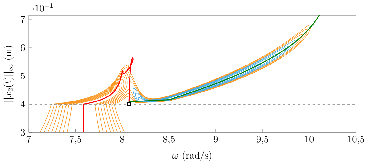
FIGURE V.10 – Première famille d'isolats, courbes de réponse principales de A = 1 à A = 2,4 par pas de 0,2 (—), isolats A = 1 à A = 1,8 par pas de 0,2 (—), NNM 1 (—), NNM 5 (—), g_0 (—), premier point singulier (■).
