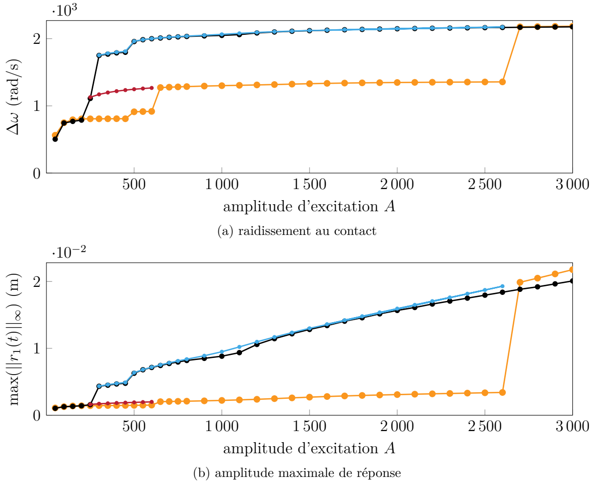
FIGURE V.34 – Évolution de la position de la résonance non linéaire en fonction de A pour l'aube rotor 37, courbe de réponse principale (—○—), prédiction du principe énergétique de Melnikov (—●—), première famille d'isolats (—●—), seconde famille d'isolats (—●—).
