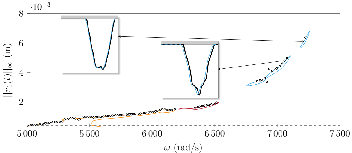
FIGURE V.33 – Validation des solutions de la DLFT-HBM pour A = 550 sur le rotor 37, courbe de réponse principale (—), branches de solutions isolées (—) (—), solutions IT ( \bullet ), c_1 (—).
