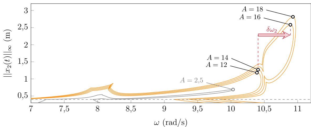
FIGURE V.4 – Deuxième discontinuité de la résonance non linéaire par rapport à A , courbe de réponse avec A \in \{12; 14; 16; 18\} (—), courbe de réponse avec A \in \{2,5\} (—), g_0 (---), résonances non linéaires (o) (o).
