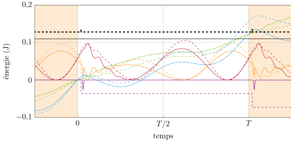
FIGURE IV.8 – Bilan énergétique sur une période pour m_2 = 2 \text{ kg} ( N_t = 4000 ), IT (---), DLFT-HBM (—), énergie totale (■), énergie cinétique (■), énergie potentielle (■), énergie dissipée (intégrale) (■), travail des efforts d'excitation (intégrale) (■), travail des efforts de contact (intégrale) (■).
