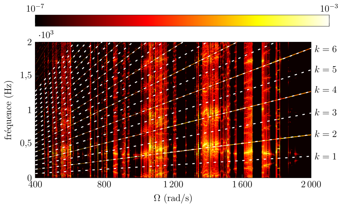
FIGURE IV.42 – Carte d'interaction obtenue par IT pour le déplacement radial du bord d'attaque, ordre moteur f = k\Omega avec k \in \mathbb{N}^* (—).
