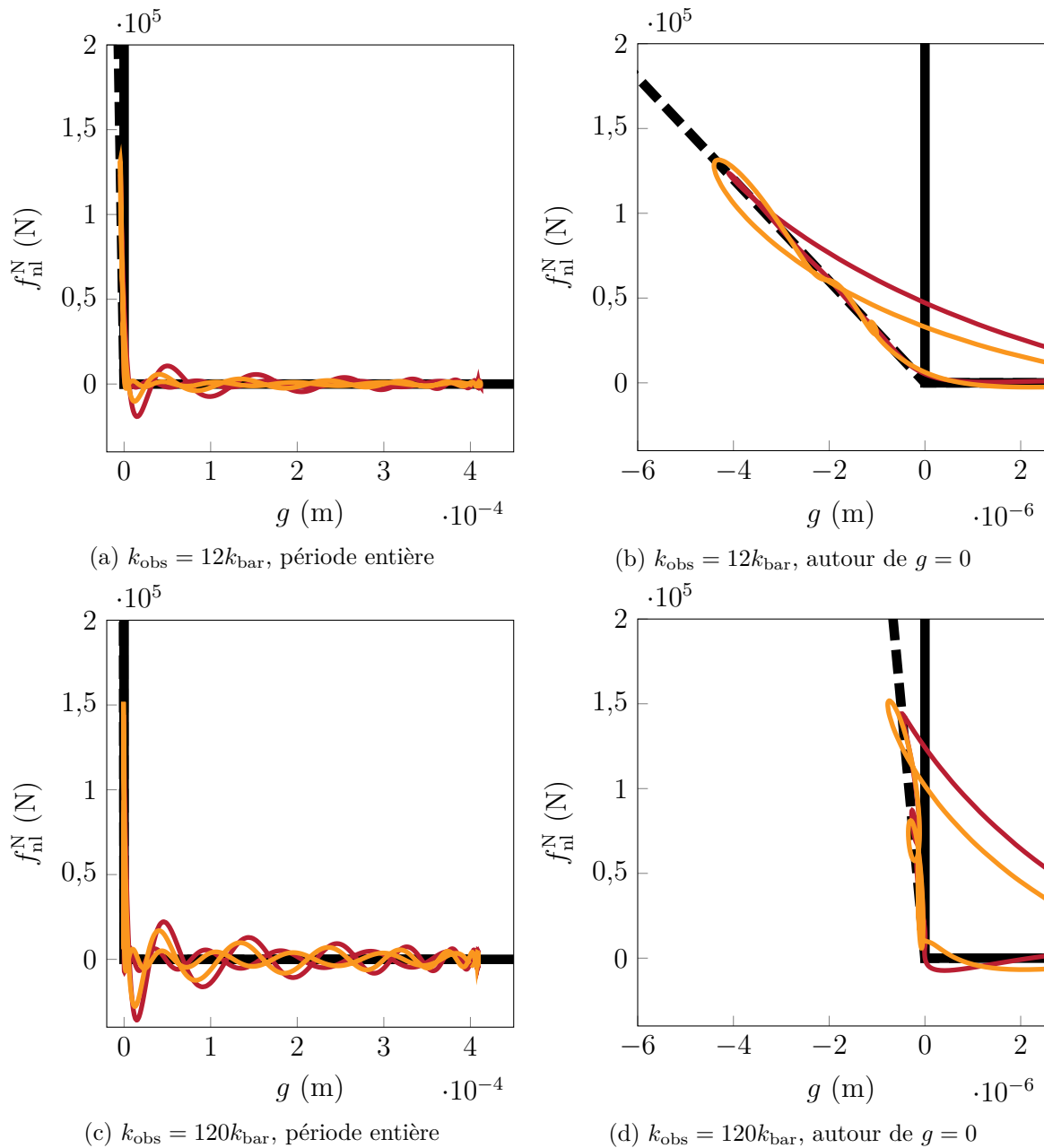
FIGURE IV.27 – Lois de contact simulées pour un obstacle rigide avec pénalité bilinéaire à différentes valeurs de k_{\text{obs}} pour N_{\text{h}} = 20 et N_{\text{t}} = 400 à \omega = \omega_1 , DLFT-HBM (—), LCP-HBM (—), loi de pénalité f_{\text{nl}}^{\text{N}} = \max(-k_{\text{obs}}g, 0) (---), contact unilatéral (—).
