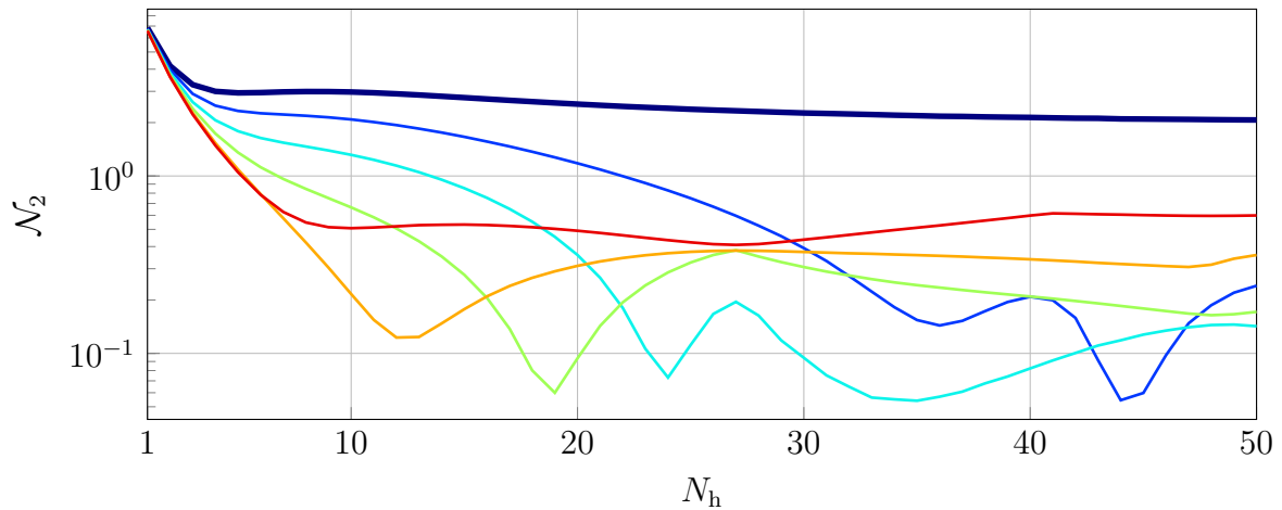
FIGURE IV.14 – Evolution de \mathcal{N}_2 en fonction de N_h ( N_t = 2000 et m_2 = 2 kg, \omega = 0,9 \text{ rad}\cdot\text{s}^{-1} ), n_{\text{dep}} = 0\% (DLFT-HBM classique) (—), n_{\text{dep}} = 1\% (—), n_{\text{dep}} = 2\% (—), n_{\text{dep}} = 3\% (—), n_{\text{dep}} = 4\% (—), n_{\text{dep}} = 5\% (—).
