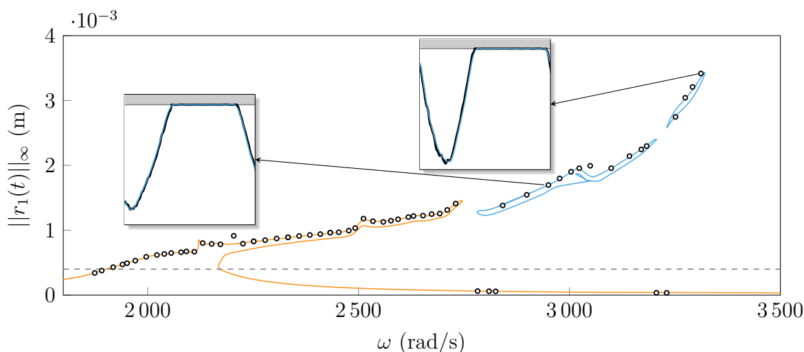
FIGURE V.40 – Validation des solutions de la DLFT-HBM par IT pour A = 140 , courbe de réponse principale (—), branches de solutions isolées (—), IT ( \circ ), c_1 (—). Graphes de déplacements : DLFT-HBM (—), IT (—), carter (■).
