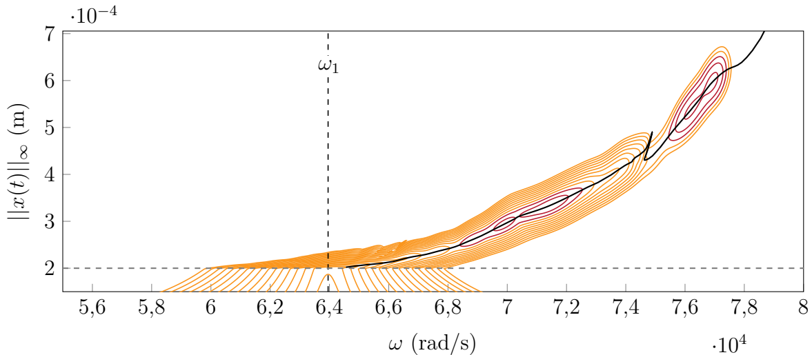
FIGURE V.26 – Suivi de points limites pour la barre éléments-finis, vue 2D, courbes de réponse principales (—), branches de solutions isolées (—), points limites (—), g_0 (- -).
