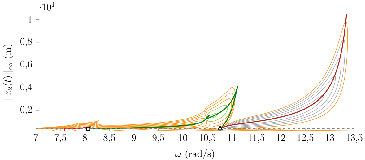
FIGURE V.15 – Troisième famille d'isolats, courbes de réponse principales de A = 5 à A = 30 par pas de 5 (—), branches isolées (famille 2) pour A = 10 et A = 15 (—), branches isolées (famille 3) de A = 5 à A = 25 par pas de 5 (—), NNM 1 (—), NNM 5 (—), NNM 6 (—), g_0 (—), premier point singulier (□), second point singulier (Δ).
