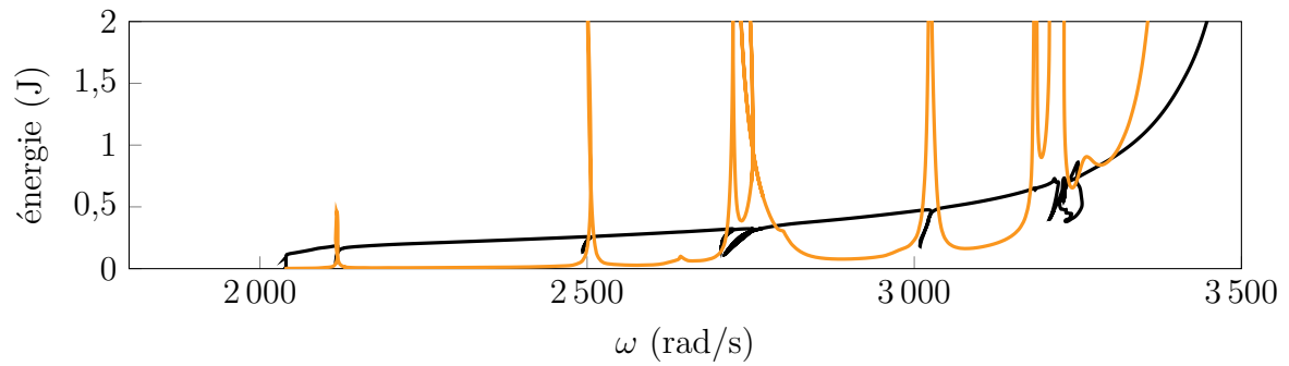
FIGURE V.38 – Principe énergétique de Melnikov pour A = 140 sur le rotor 67, résistance |\mathcal{R}_{in}| + |\mathcal{R}_{nl}| (—), terme de travail |W^{1:1}| (—).
