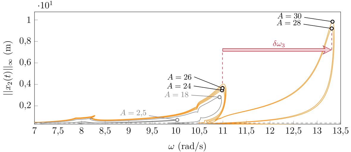
FIGURE V.5 – Troisième discontinuité de la résonance non linéaire par rapport à A , courbe de réponse avec A \in \{24; 26; 28; 30\} (—), courbe de réponse avec A \in \{2,5; 18\} (—), g_0 (---), résonances non linéaires (o) (o).
