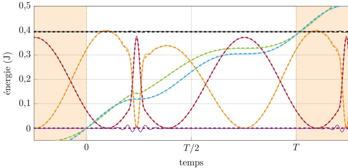
FIGURE IV.6 – Bilan énergétique sur une période pour m_2 = 0 kg, IT (••), DLFT-HBM (—), énergie totale (■), énergie cinétique (■), énergie potentielle (■), énergie dissipée (intégrale) (■), travail des efforts d'excitation (intégrale) (■), travail des efforts de contact (intégrale) (■).
