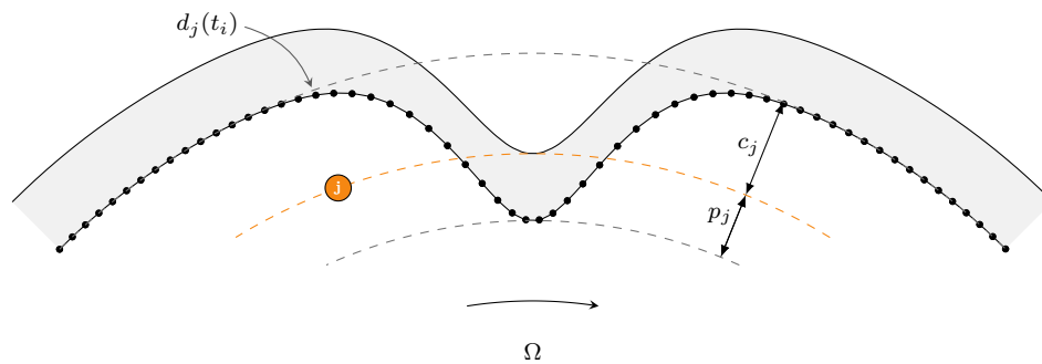
FIGURE IV.39 – Déformation à un lobe du carter ( \square ) en face du j -ième nœud frontière ( \bullet ).
