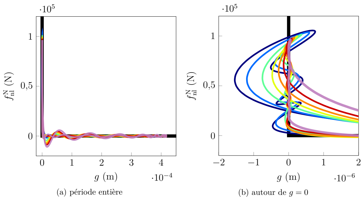
FIGURE IV.33 – Étude paramétrique sur les lois de contact en fonction de \varepsilon pour N_h = 20 , N_t = 600 et k_{obs} = 4k_{bar} à \omega = \omega_1 , LCP-HBM (—), DLFT-HBM (—), contact unilatéral (—).
