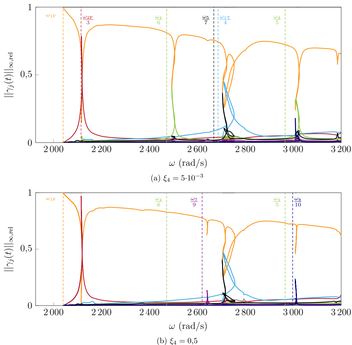
FIGURE V.45 – Contributions modales relatives le long des NNM pour deux taux d'amortissement \xi_4 , 1F mode (—), mode 2F (—), mode 1T (—), quatrième mode (—), cinquième mode (—), septième mode (—), huitième mode (—), autres modes (—).
