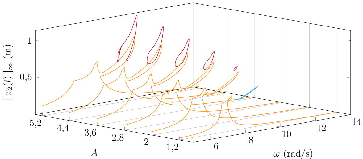
FIGURE V.21 – Première famille d'isolats de période double, courbes de réponse principales (—), branche de solutions isolées de période simple (—), branches de solutions isolées de période double (—), points de bifurcation (◦).
