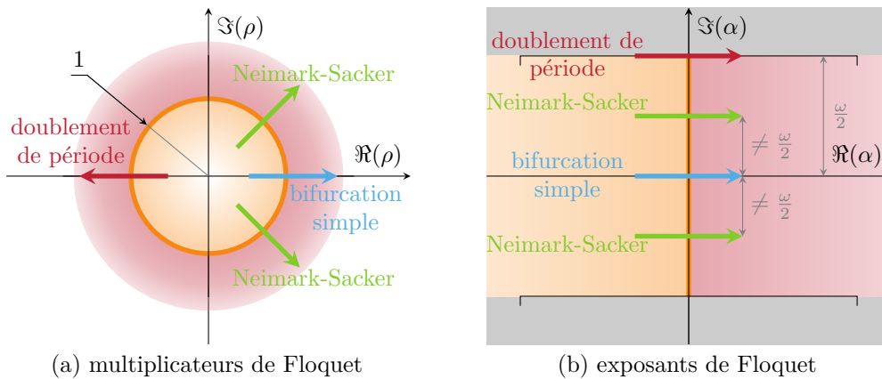
FIGURE II.9 – Bifurcations des solutions périodiques, limite de stabilité (—), zone stable (■), zone instable (■), les crochets délimitent la cellule primitive ] -\frac{\omega}{2}; \frac{\omega}{2}] , adaptée de [206, 229].
