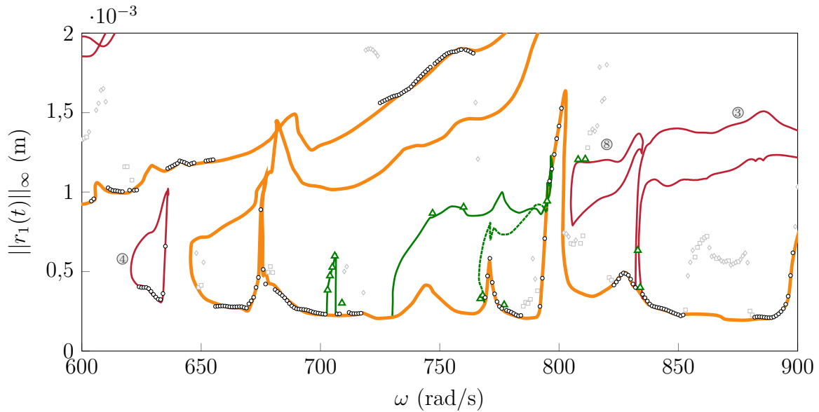
FIGURE IV.47 – Branches de période double capturées par la DLFT-HBM, courbe de réponse principale (—), branches de solutions isolées (—), branches de période double (—), (---), IT de pulsation fondamentale \omega : \omega = 2\Omega (○), \omega = \Omega (△), sous-harmonique ( \omega < \Omega ) (□), pas de périodicité ou \omega < \Omega/10 (◇).
