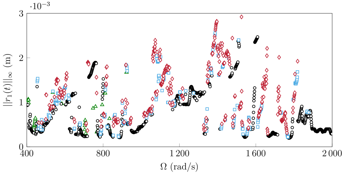
FIGURE IV.43 – Courbe de réponse en fréquence obtenue par IT au bord d'attaque, pulsation fondamentale \omega : \omega = 2\Omega ( \circ ), \omega = \Omega ( \triangle ), sous-harmonique ( \omega < \Omega ) ( \square ), pas de périodicité ou \omega < \Omega/10 ( \diamond ).
