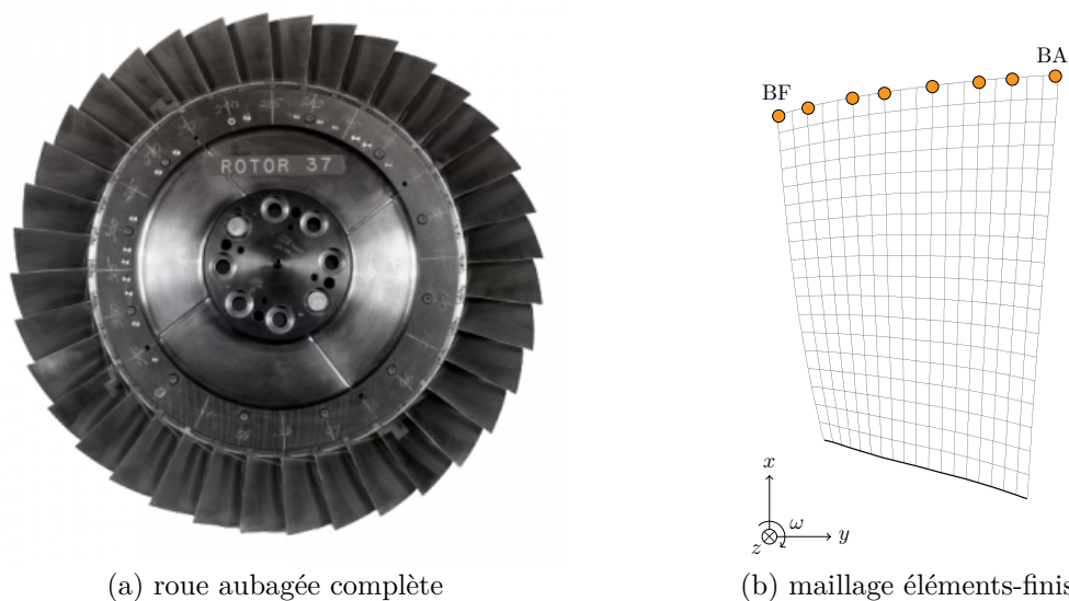
FIGURE V.28 – NASA rotor 37 [235], nœud frontière (●), encastrement (—)
