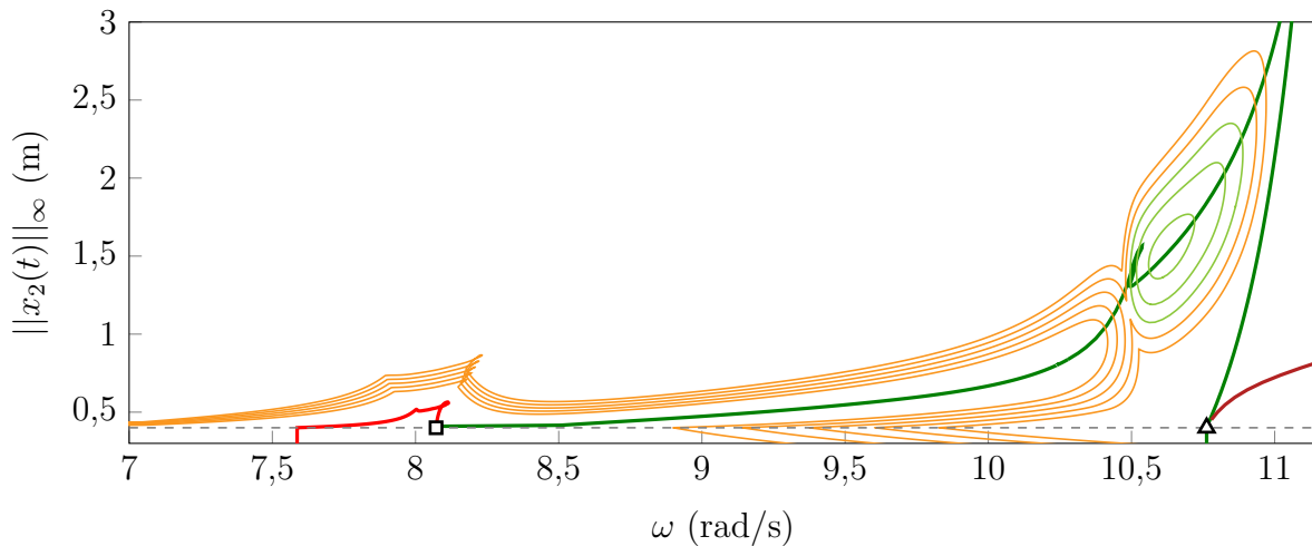
FIGURE V.13 – Deuxième famille d'isolats, courbes de réponse principales de A = 10 à A = 18 par pas de 2 (—), branches de solutions isolées de A = 10 à A = 14 par pas de 2 (—), NNM 1 (—), NNM 5 (—), NNM 6 (—), g_0 (—), premier point singulier (■), second point singulier (▲).
