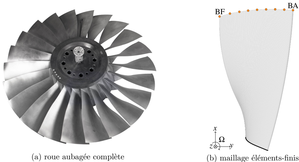
FIGURE IV.40 – NASA rotor 67 [237], nœud frontière (●), encastrement (—).
