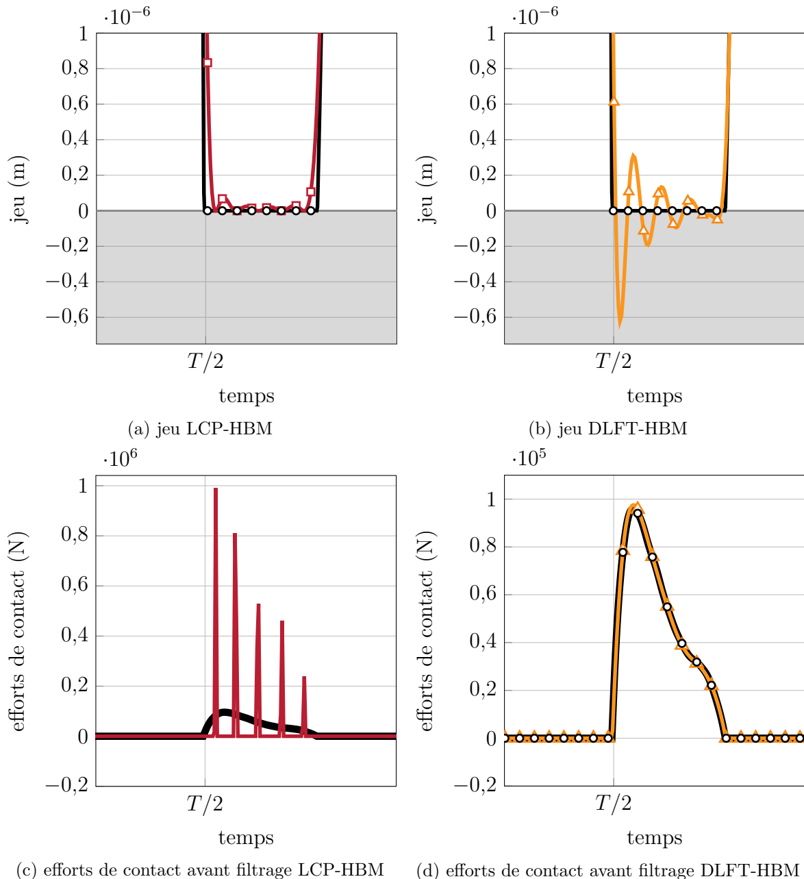
FIGURE IV.24 – Jeu et efforts de contact avant troncature pour N_h = 20 et N_t = 400 , IT (obstacle flexible) ( \bullet - \circ ), DLFT-HBM ( \blacktriangle - \blacktriangleright ), LCP-HBM ( \blacksquare - \blacktriangleright ), obstacle ( \blacksquare ).
