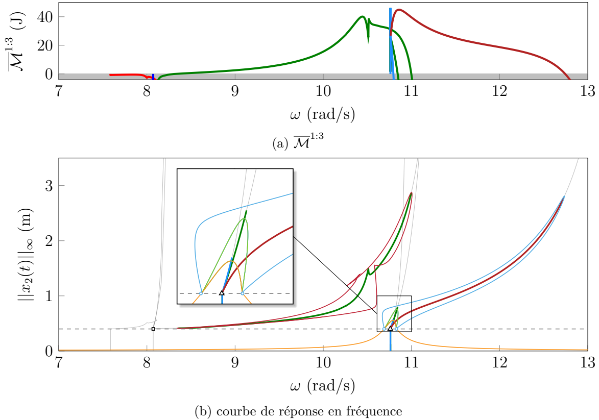
FIGURE V.25 – Analyse de Melnikov pour une excitation du deuxième mode sur la troisième harmonique avec A = 20 , NNM 5 (—), NNM 6 (—), NNM 7 (—), courbe de réponse principale (—), branche de solutions isolées et bifurquées (—) (—) (—), deux orbites périodiques persistent ( \overline{\mathcal{M}}^{1:3} > 0 ) (—), aucune orbite périodique ne persiste ( \overline{\mathcal{M}}^{1:3} < 0 ) (—), g_0 (—), premier point singulier (■), second point singulier (▲), points de bifurcation (○).
