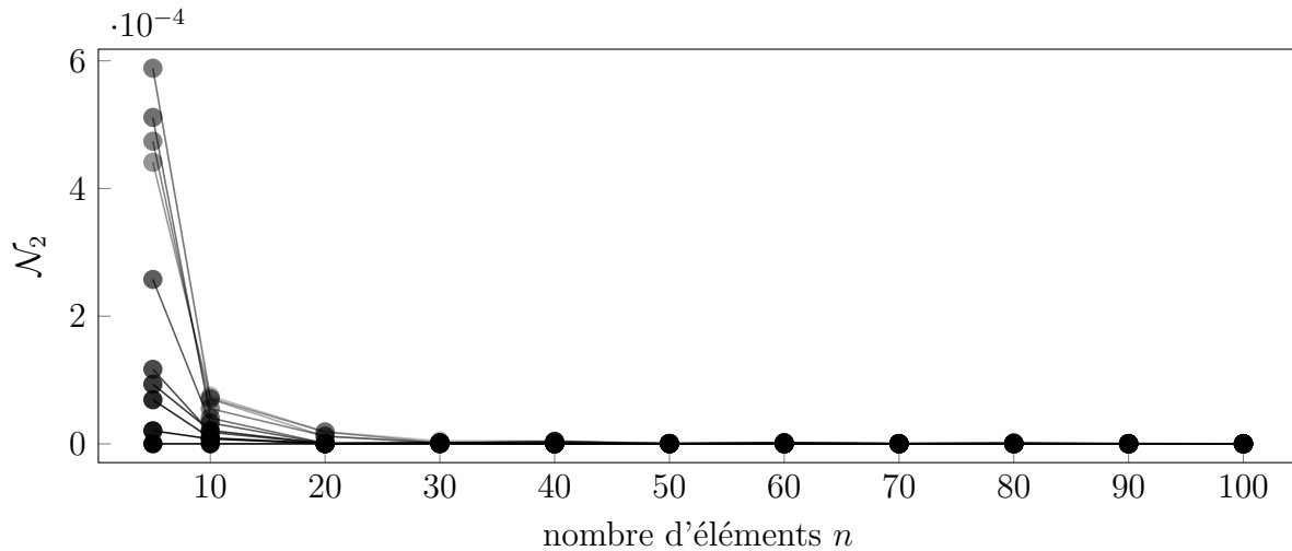
FIGURE IV.20 – Evolution de \mathcal{N}_2 en fonction du nombre d'éléments n de la barre à plusieurs coefficients de restitution e .
