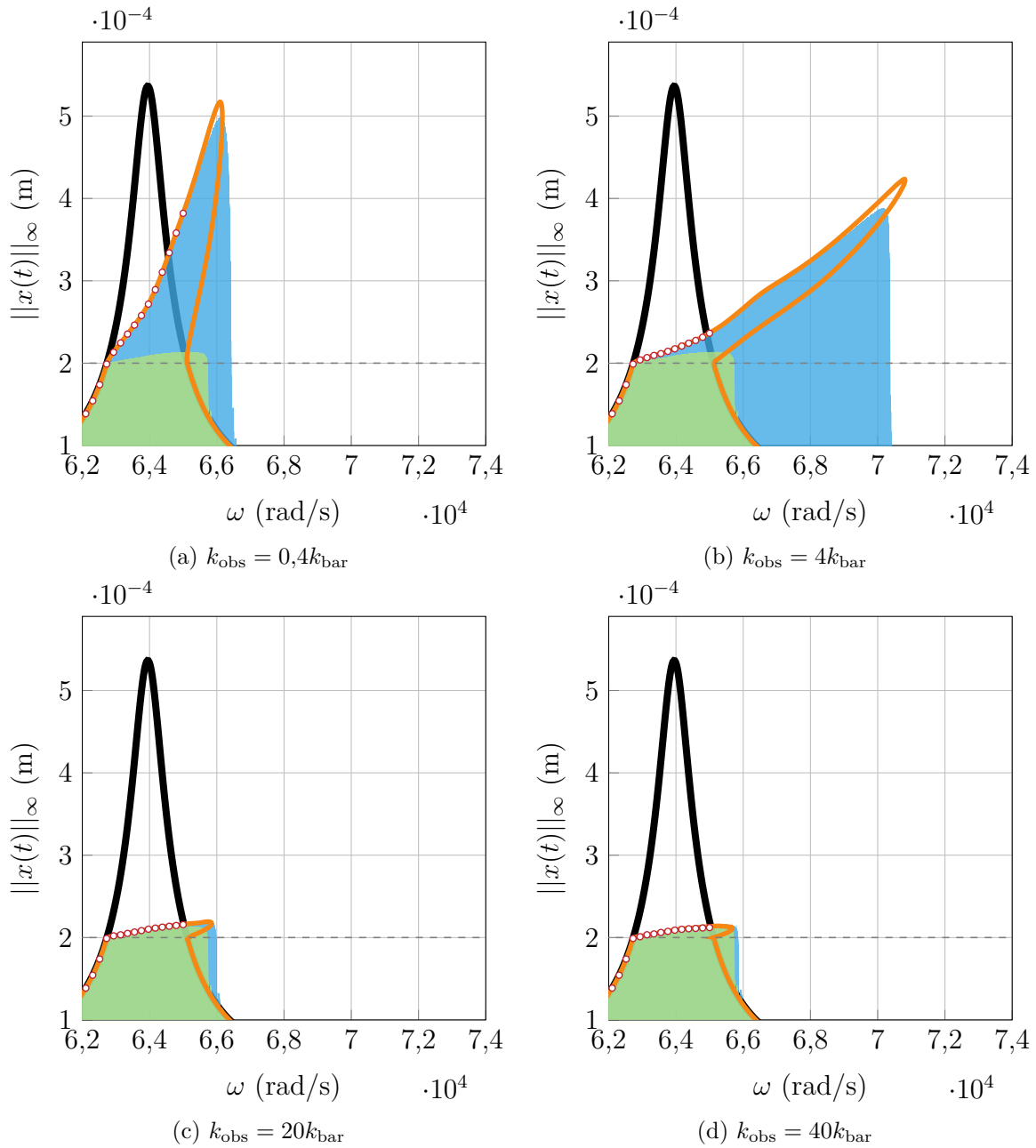
FIGURE IV.29 – Courbes de réponse en fréquence pour différentes valeurs de k_{\text{obs}} pour N_{\text{h}} = 20 et N_{\text{t}} = 400 , linéaire (—), DLFT-HBM (—), LCP-HBM ( \circ ), IT balayage linéaire (pénalité) (■), IT balayage linéaire (Lagrange) (■), g_0 (- -).
