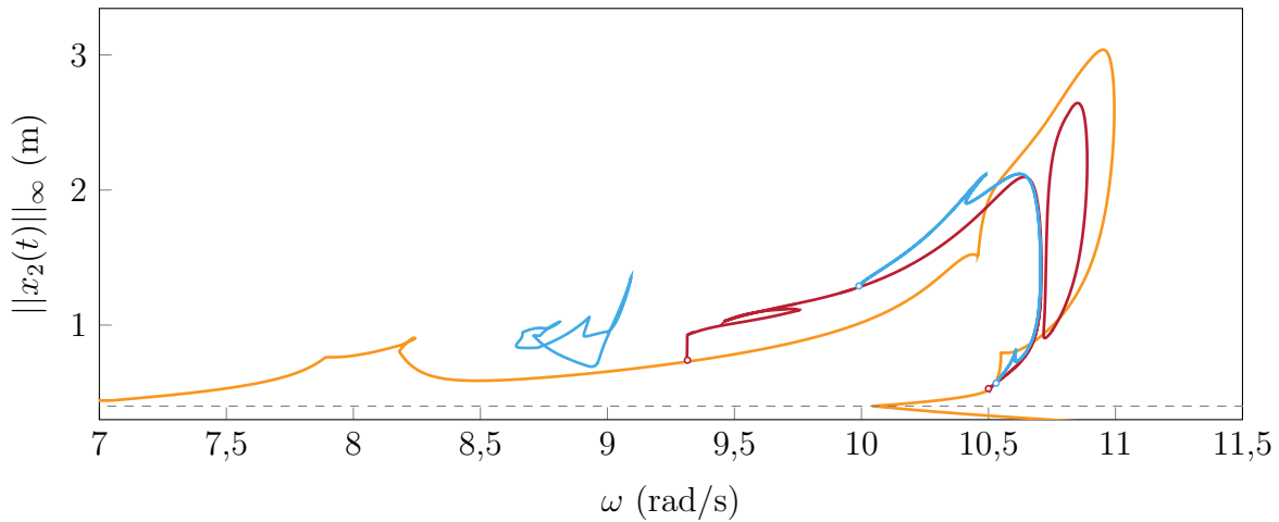
FIGURE V.20 – Branches de période double et quadruple pour A = 20 , courbe de réponse principale (—), branches de période double (—), branches de période quadruple (—), g_0 (---), points de bifurcation (◦) (◦).
