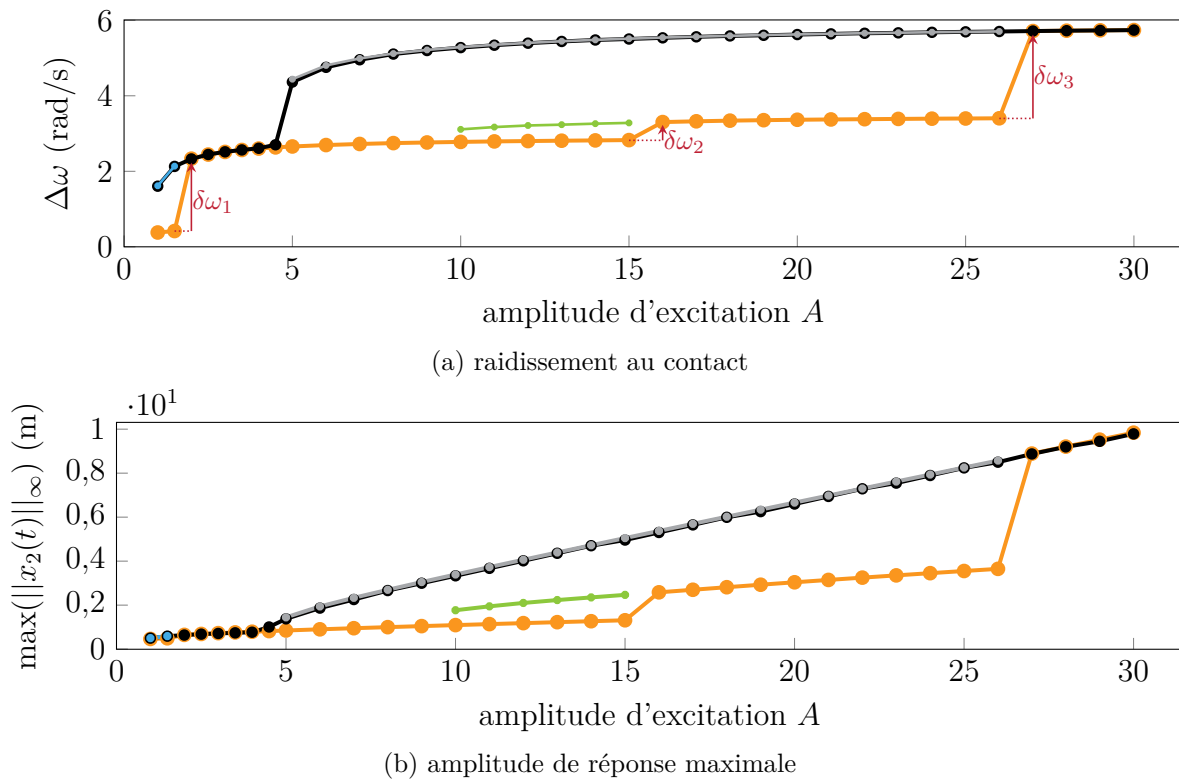
FIGURE V.16 – Évolution de la résonance non linéaire en fonction de A , courbe de réponse principale (—), prédiction du principe énergétique de Melnikov (—), première famille d'isolats (—), deuxième famille d'isolats (—), troisième famille d'isolats (—).
