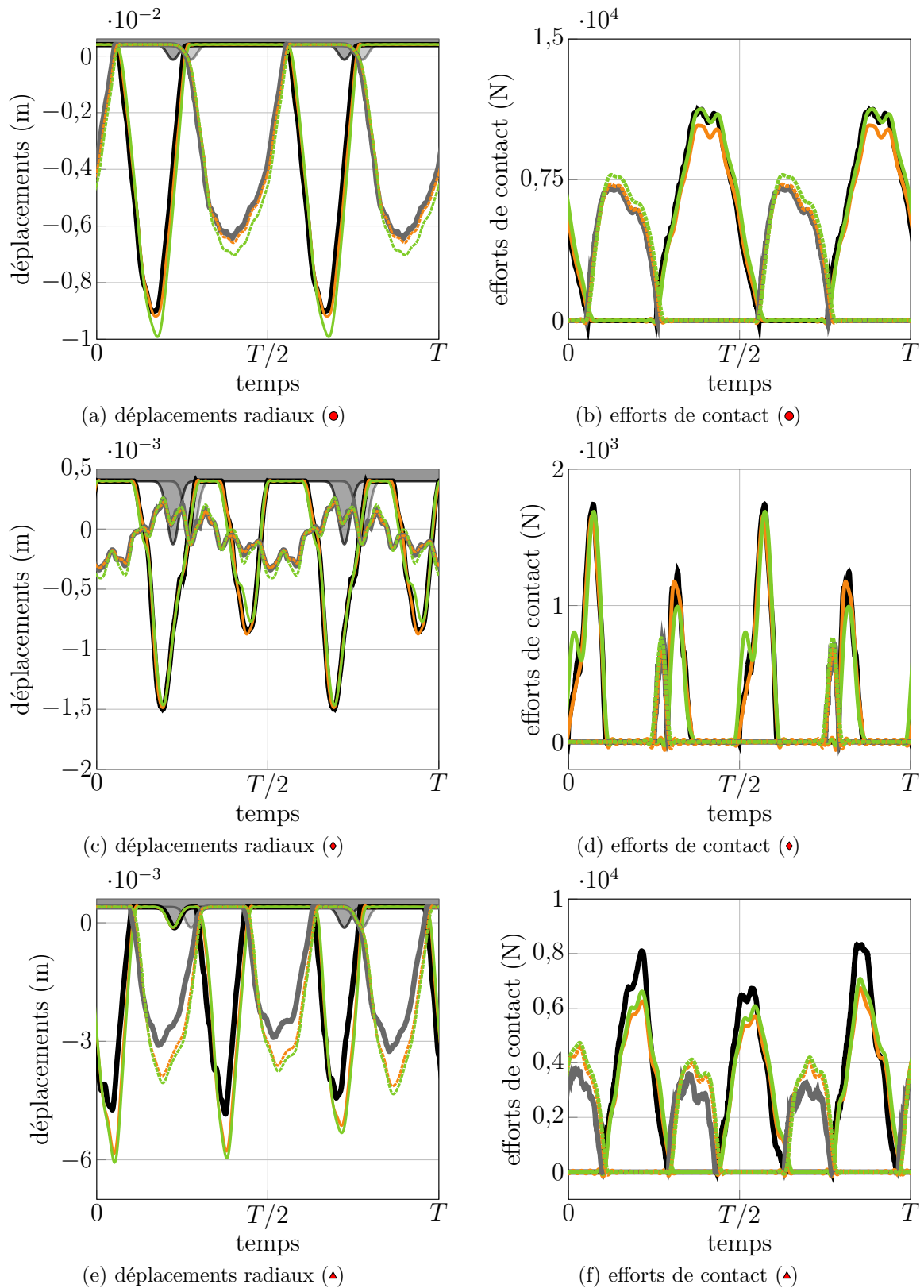
FIGURE IV.48 – Signaux temporels de déplacements radiaux et d'efforts de contact à la résonance principale ( \bullet ), sur l'isolat ① ( \blacklozenge ) et la branche ③ ( \blacktriangle ), DLFT-HBM : BA (—) BF (—), RL-HBM : BA (—) BF (—), IT : BA (—) BF (—).
