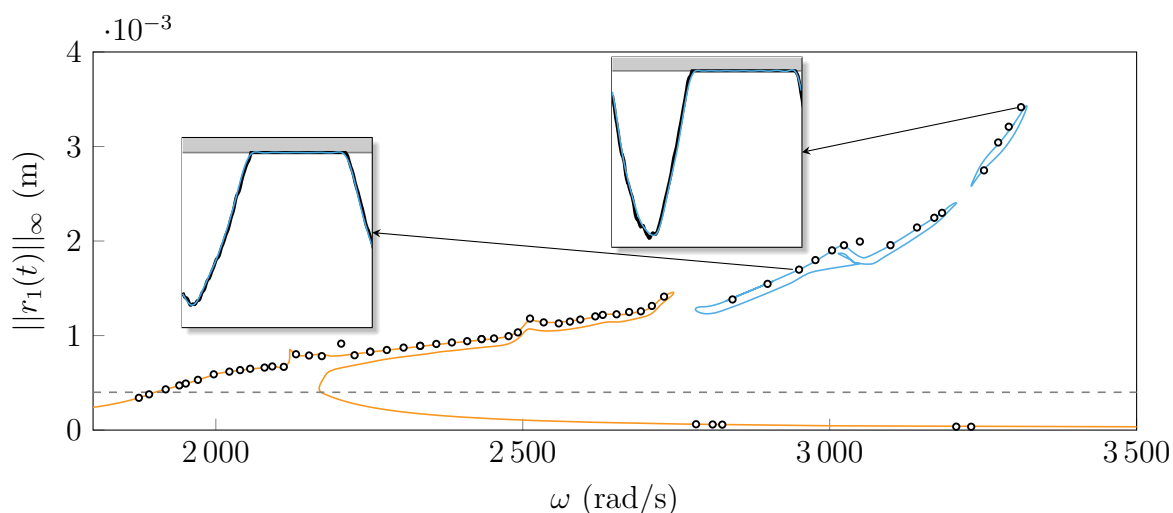
FIGURE V.40 – Validation des solutions de la DLFT-HBM par IT pour A = 140 , courbe de réponse principale (—), branches de solutions isolées (—), IT ( \circ ), c_1 (- -). Graphes de déplacements : DLFT-HBM (—), IT (—), carter (■).
