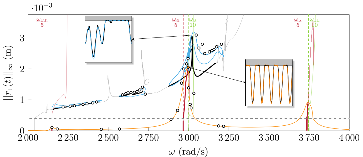
FIGURE V.49 – Analyse de Melnikov pour une forme d'excitation aléatoire sur le cinquième harmonique avec A = 50 \|\mathbf{M}\Phi_{1T}\| , courbe de réponse principale (—), NNM 1F (—), NNM surharmoniques de pulsation fondamentale 5\omega (—) et 10\omega (—), branches de solutions isolées (—), deux orbites périodiques persistent ( \overline{\mathcal{M}}^{1:5} > 0 ) (—), aucune orbite périodique ne persiste ( \overline{\mathcal{M}}^{1:5} < 0 ) (—), c_1 (—), simulations IT (o).
