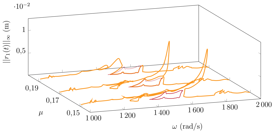
FIGURE IV.54 – Etude d'influence sur le coefficient de frottement \mu , courbe de réponse principale (—), isolat ④ ( \mu = 0,15 ) ④ (—), isolat ④ projeté sur les plans \mu = 0,17 et \mu = 0,19 (.....).
