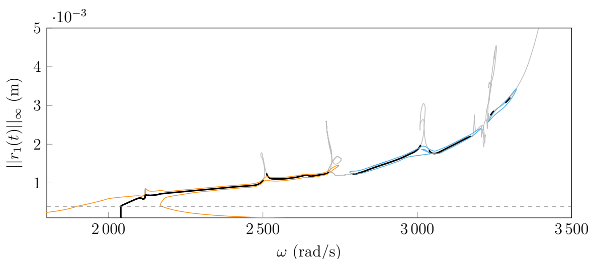
FIGURE V.39 – Réponse en fréquence du rotor 67 pour A = 140 , courbe de réponse principale (—), branches de solutions isolées (—), NNM 1F (—), deux orbites périodiques persistantes ( \overline{\mathcal{M}}^{1:1} > 0 ) (—), aucune orbite périodique ne persiste ( \overline{\mathcal{M}}^{1:1} < 0 ) (—), c_1 (- -).
