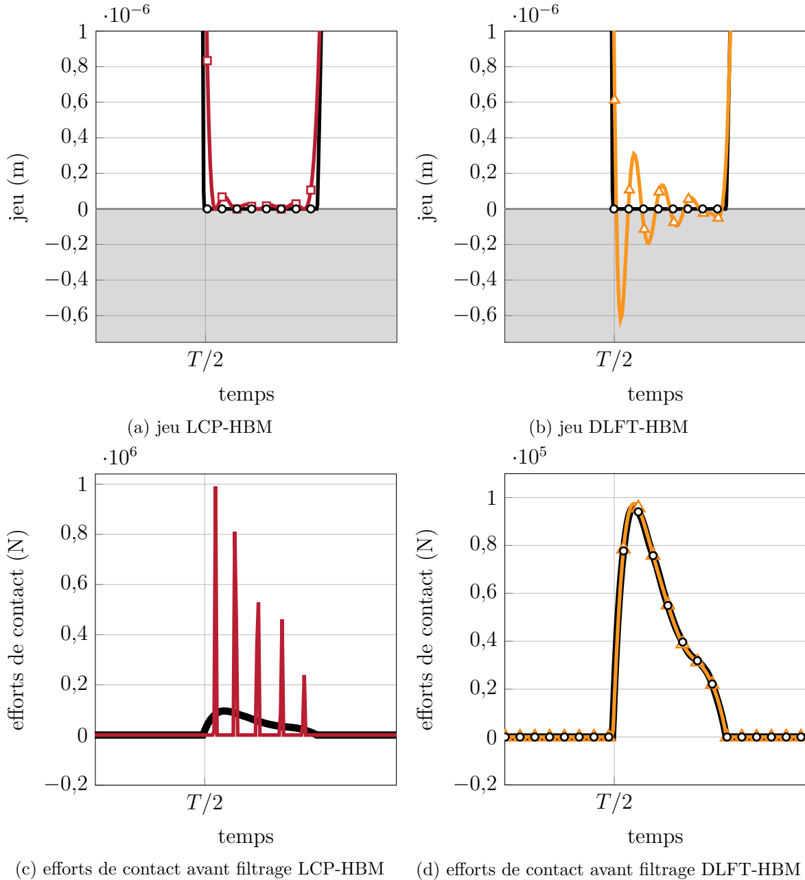
FIGURE IV.24 – Jeu et efforts de contact avant troncature pour N_h = 20 et N_t = 400 , IT (obstacle flexible) ( \bullet - \circ ), DLFT-HBM ( \blacktriangle - \blacktriangleright ), LCP-HBM ( \square - \square ), obstacle ( \square ).
