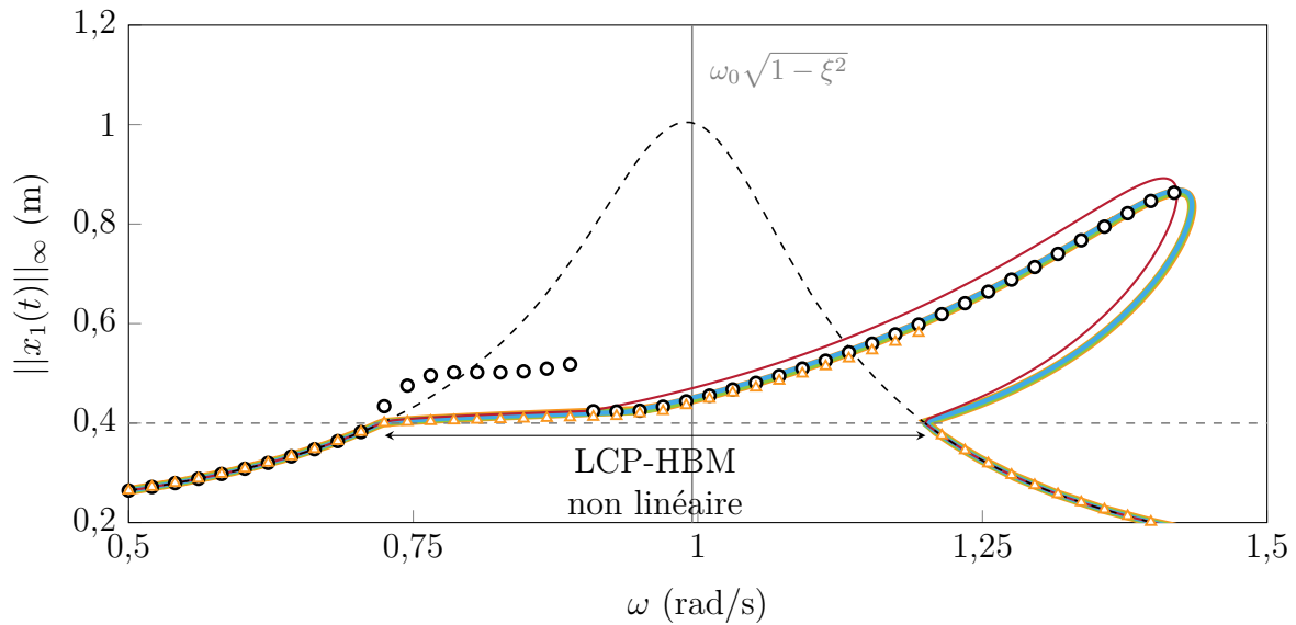
FIGURE IV.2 – Convergence de la réponse en fonction du nombre d'harmoniques autour de la fréquence de résonance (—), réponse linéaire (- -), g_0 (- -), LCP-HBM N_h = 40 ( \Delta ), IT ( \circ ), DLFT-HBM : N_h = 10 (—), N_h = 20 (—), N_h = 30 (—), N_h = 40 (—).
