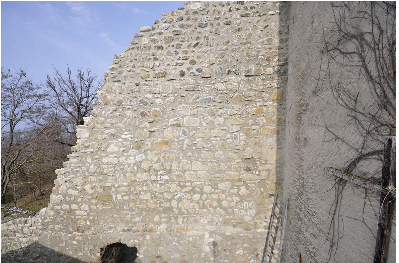
Fig. 16: Mur bouclier de Château-Neuf après restauration. Cliché : L. Benoit.
