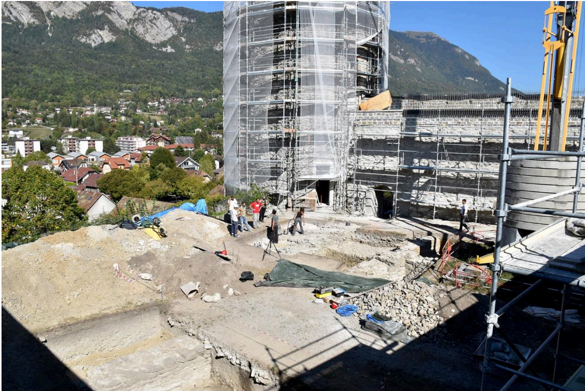
Fig. 6: Vue de la courtine orientale depuis l'intérieur du château. Cliché : L. Benoit.
