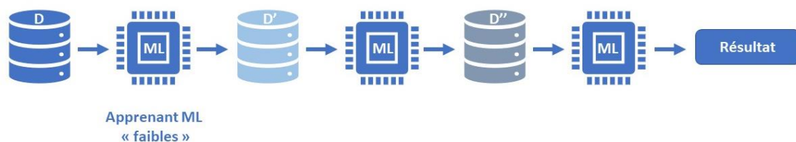
Figure 14: Schéma de fonctionnement du Boosting. Cette méthode attribue des poids aux prédictions fausses pour que les apprenants suivants se focalisent sur ces données.
