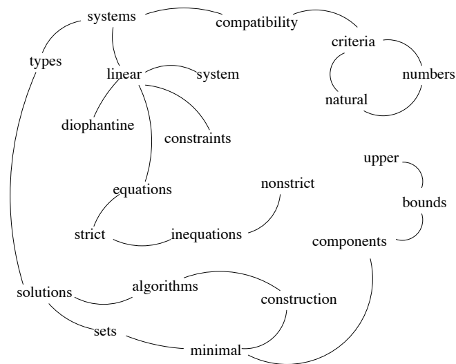
FIGURE 2.1. – Exemple de document de la collection de test Inspec (Hulth, 2003) (docid: 1939.abstr) et de sa représentation en graphe de cooccurrences de mots reprises de l'article de TextRank (Mihalcea and Tarau, 2004). Les mots-clés extraits par TextRank (i. e. séquences contiguës des mots les plus importants) sont marqués en rouge dans le texte.
