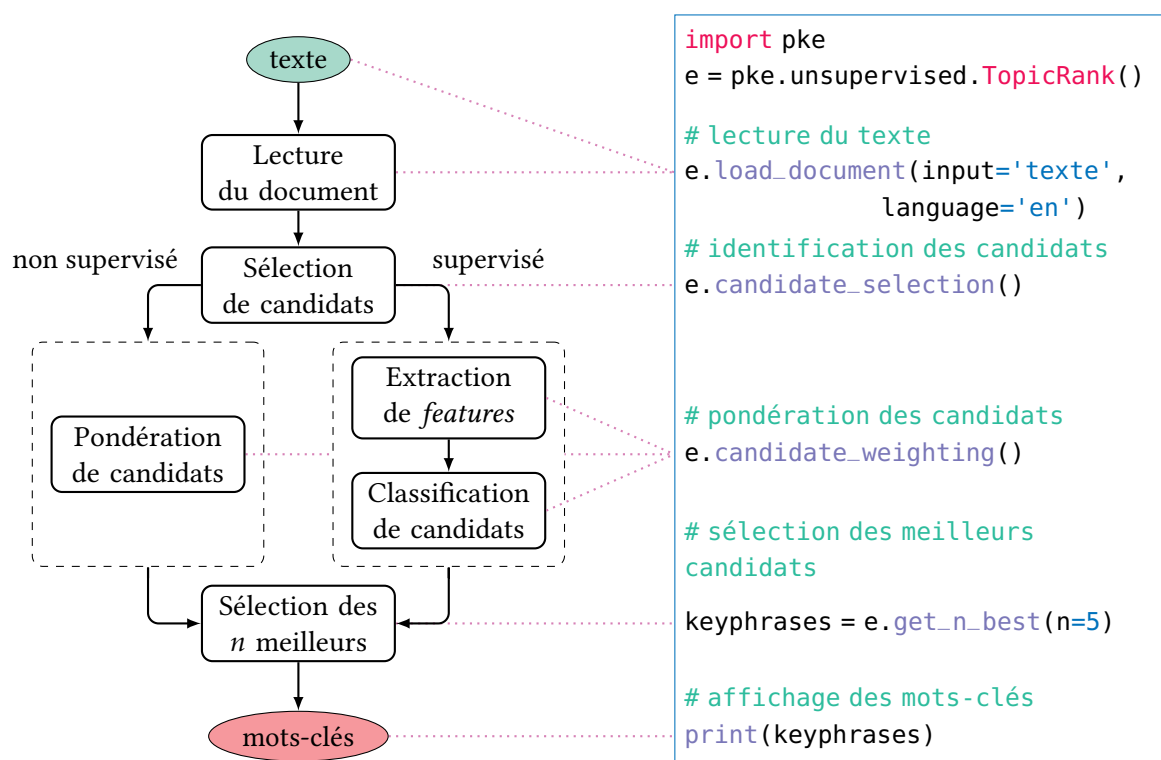
FIGURE 5.1. – Architecture de la bibliothèque logicielle pke (à gauche) associée à un exemple minimal d’utilisation de son API (à droite).
