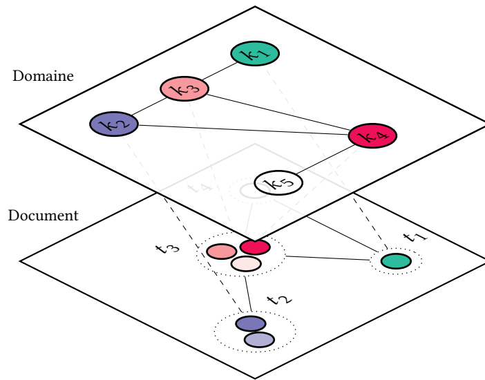
FIGURE 2.4. – Illustration du modèle TopicCoRank qui unifie les représentations en graphe du domaine (mots-clés de référence) et du document (sujets).
