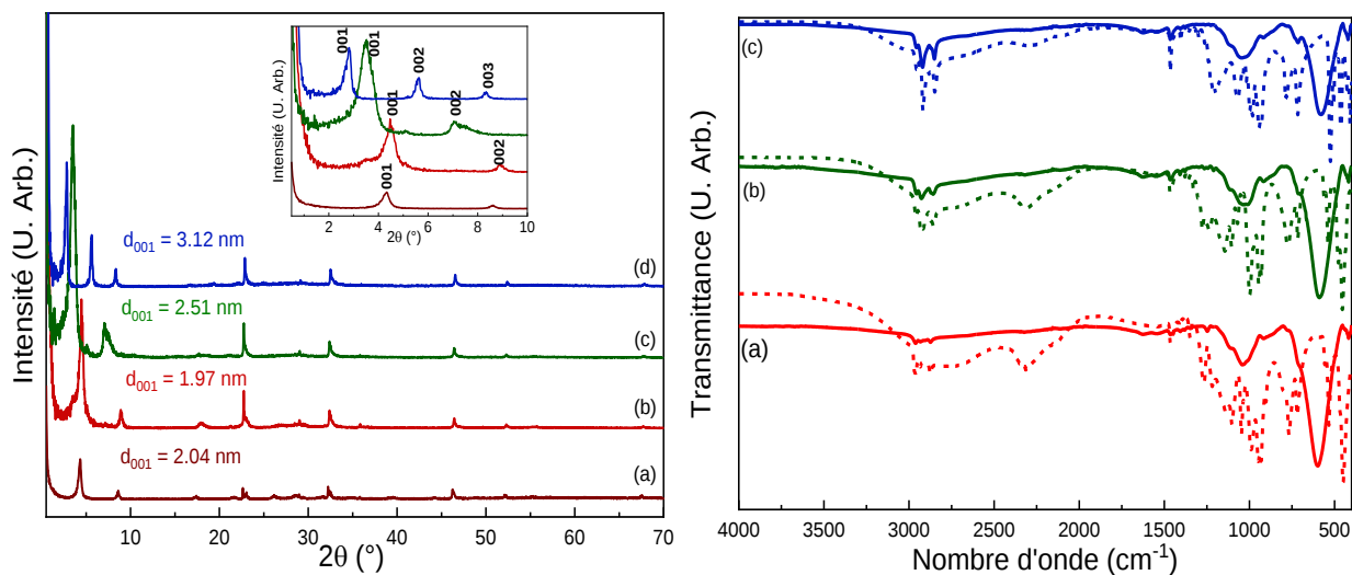
Figure 2: Gauche) Diffractogrammes (a) du précurseur C_4N -HST, (b) C_3PO_3 -HST (c) C_6PO_3 -HST et (d) C_{10}PO_3 -HST Droite) Spectres FTIR de (a) C_3PO_3 -HST (b) C_6PO_3 -HST et (d) C_{10}PO_3 -HST en ligne pleine et les dérivés d'acide phosphonique correspondants en pointillés.
