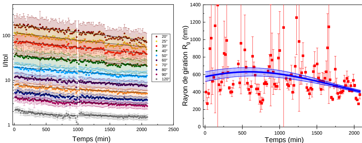
Figure 13: (Gauche) Evolution temporelle de l'intensité diffusée à plusieurs angles de diffusion. Les lignes noires correspondent à l'interpolation en utilisant un fit exponentiel. (Droite) Evolution temporelle rayon de giration apparent. La ligne continue bleue correspond aux valeurs obtenues avec un fit exponentiel tandis que les carrés rouges sont obtenus à partir d'un fit parabolique.
