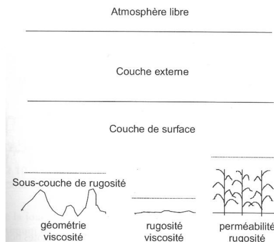
Fig. n°20 Représentation schématique des différentes parties de la couche limite planétaire. (Guyot, 2013 adaptée de Brutsaert, 1982).
