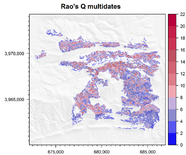
Fig.n°54 : Cartes de l'entropie quadratique de Rao. A et B : Indices monodates, C : Indice multirates.
