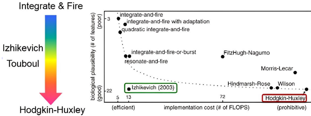
FIGURE 2.12 – Classement des différents modèles suivant le coût en calcul nécessaire afin d’être simulés et leur plausibilité par rapport à la biologie. La figure provient de www.izhikevich.com .
