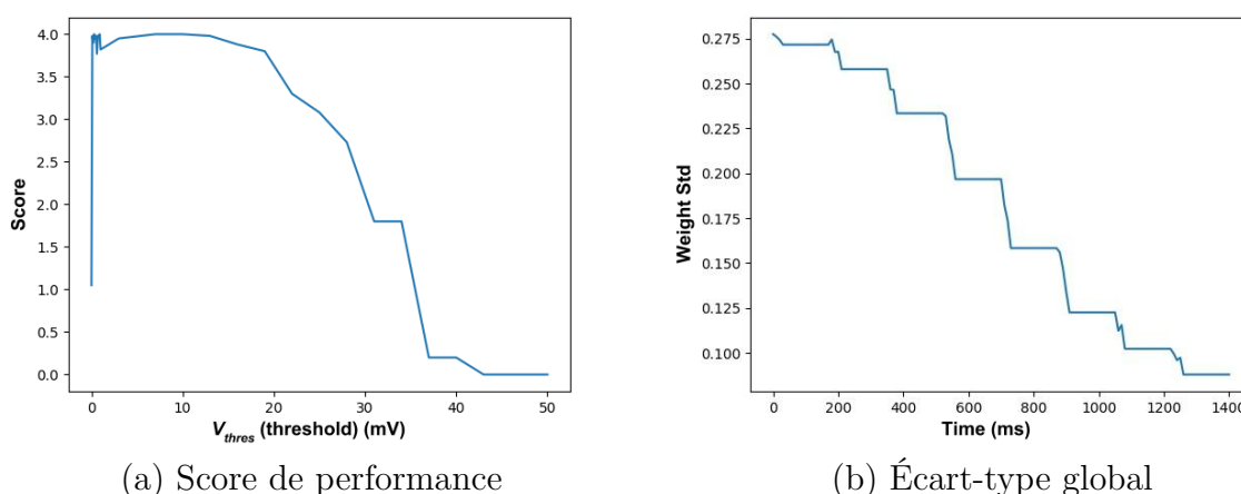
FIGURE 4.20 – Dans la figure (a), la courbe symbolisant l'évolution du score lorsque le paramètre V_{thres} varie. Dans la figure (b), la courbe symbolisant l'évolution de l'écart-type global des poids synaptiques au cours d'une simulation (cas non idéal). Les plateaux correspondent aux différentes phases de test, où la règle d'apprentissage STDP est désactivée.
