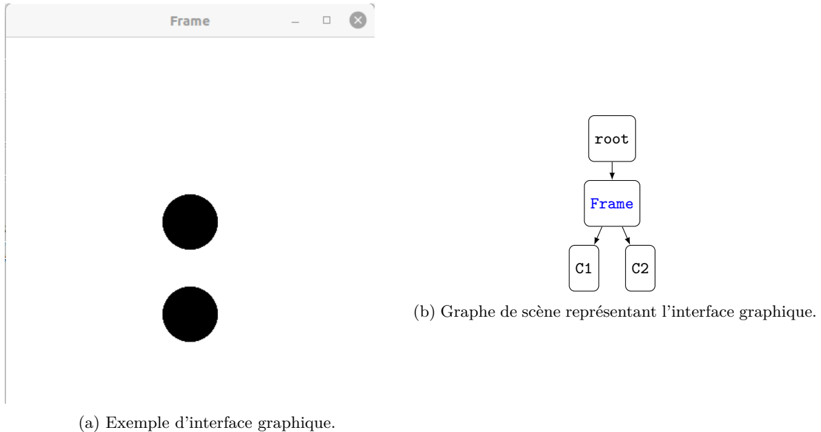
FIGURE 2.1 – Interface graphique ainsi que son graphe de scène.
