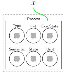
FIGURE 4.4 – Bigraphe correspondant à la sémantique structurelle d’un PROCESSUS.
