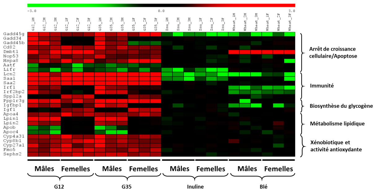
Figure 1.1. Heatmap représentant les profils d'expression génique dans le tissu hépatique des souris après un régime alimentaire supplémenté en farine de chicorée, inuline et farine de blé. Le Log2 ratio de l'expression génique est représenté pour chaque souris (1-3), les processus physiologiques associés sont représentés sur la partie droite du graphique. G12, G35: farines de chicorée.
