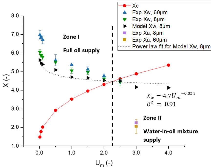
Figure 8: Comparaison entre la position X_w des gouttes d'eau obtenue expérimentalement et numériquement pour des tailles de gouttes de 8 \mu m et 60 \mu m et la position critique X_c du ménisque du contact sous-alimenté lubrifié à l'huile pure. X_a la position la plus proche de la zone de contact influencée par le ménisque air-huile
