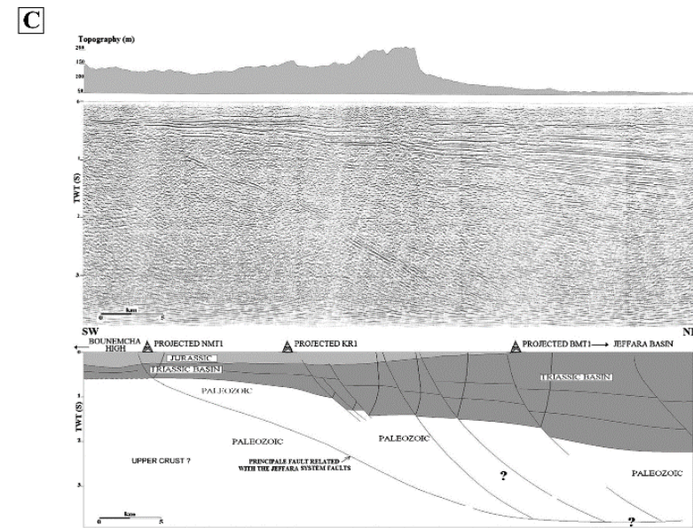
Fig. 20 (A)-Modèle régional de la croûte en Tunisie d'après les données gravimétriques (Mickus et Jallouli, 1999 ; in Gabtni, 2006) ;
