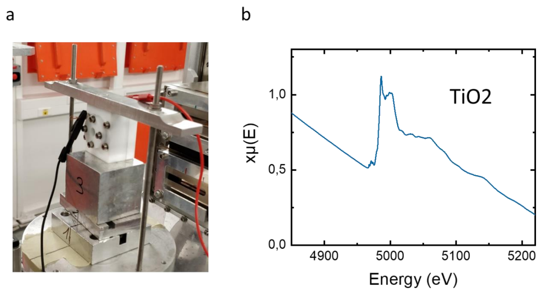
Figure 0-6 a. photos de la face arrière d'un échantillon, on peut y distinguer les 5 membranes gravées, ainsi que les dimensions de l'échantillon schématisées. b. Vue en coupe d'une membrane au MEB. c. schéma de la préparation des échantillons, la photo présente un échantillon Si/Al 2 O 3 /Cr-Pt/TiO 2 3μm. d. Photo de la cellules XAS en place sur la ligne de lumière ROCK . e. spectres du TiO 2 brut résultant d'une mesure en transmission sur la cellule montée en condition de cyclage électrochimique).
