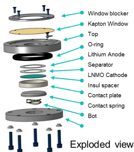
Figure 0-4 Vue explosée et photo d'un prototype en inox de la cellule électrochimique conçu dans l'objectif de réaliser des analyses operando XRD sur notre Rigaku SmartLab.
