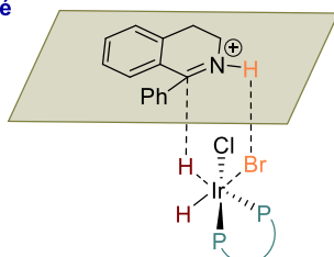
Figure 137 : Hydrogénation asymétrique de 1-aryldihydroisoquinolines
