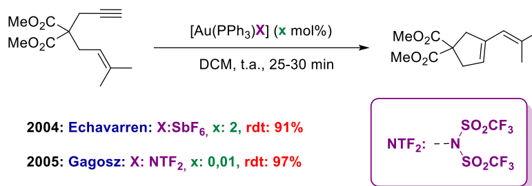
Figure 162 : Impact du contre-anion pour une réaction de cycloisomérisation d'ényne-1,6
