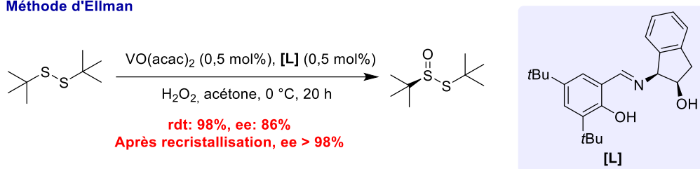
Figure 68 : Synthèse du tert -butylthiosulfinate par la méthode d'Ellman
