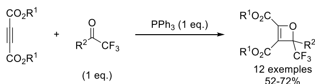
Schéma II-30 : Exemples de métathèses alcyne-carbonyle, catalysées par une phosphine pour l'accès à des oxétènes stables
