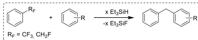
Schéma I-23 : Sélection de réactions pour lesquelles les cations fluorophosphoniums présentent une activité catalytique
