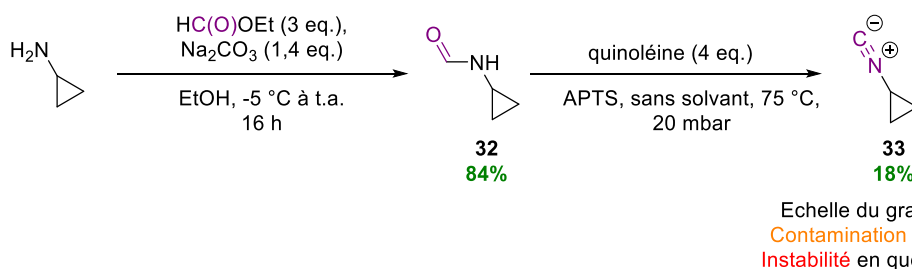
Schéma III-22 : Préparation de l'isonitrile 33 par déshydratation du formylcyclopropane, méthode de Hertler et Corey.
