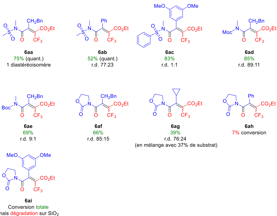
Schéma II-40 : Cycloaddition (2+2) entre les ynamides et le trifluoropyruvate d'éthyle menant aux acrylamides acycliques
