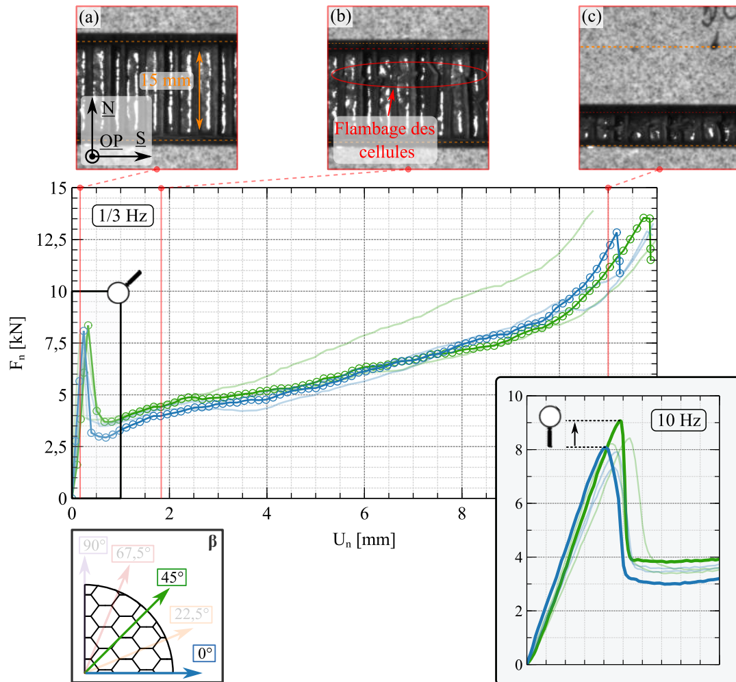
Figure 3.5 – Comportement mécanique du nid d'abeille Nomex ® HRH-10-3.2-48 sous sollicitation de compression libre.
